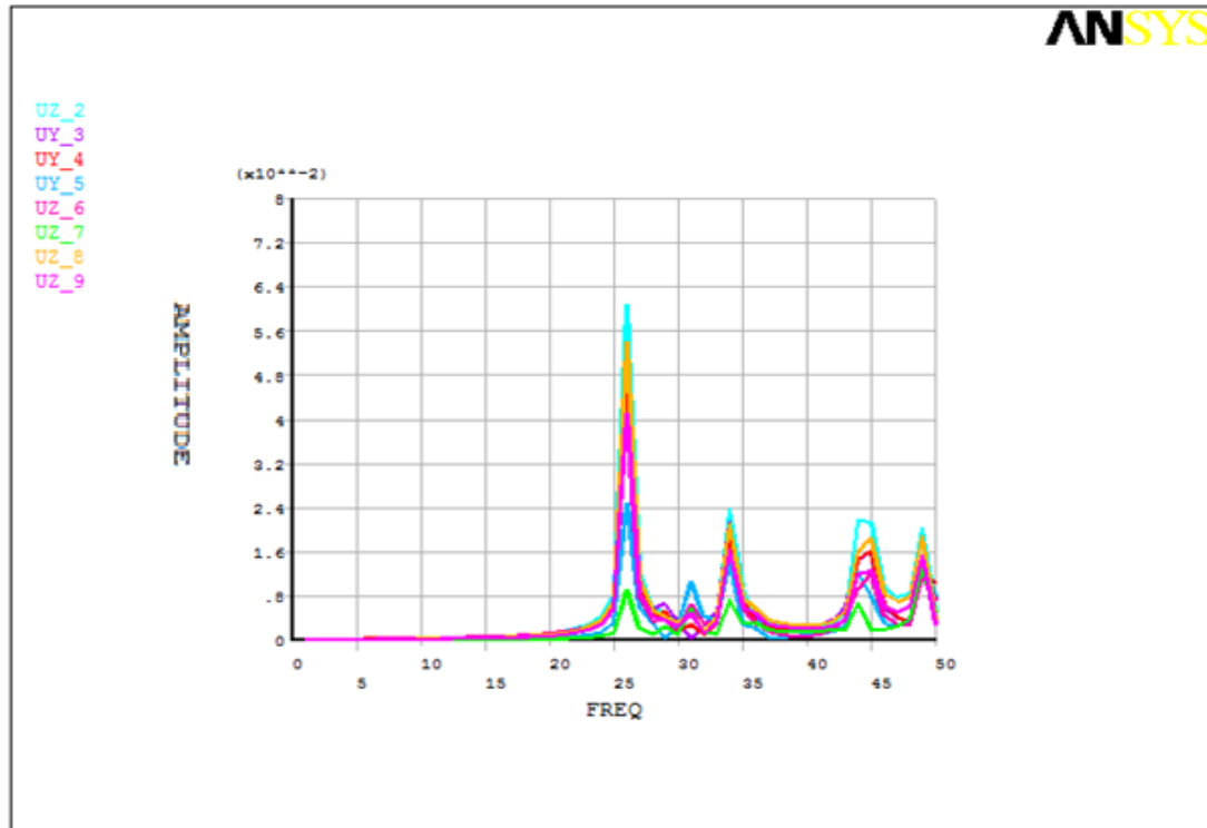
Figure 5.14 : Graphe de la repense fréquentielle cas N° 3 (acier).
