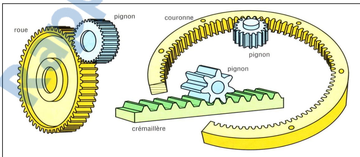
Figure 2.2 : Schéma d'engrenage (roue et pignon). [5]
