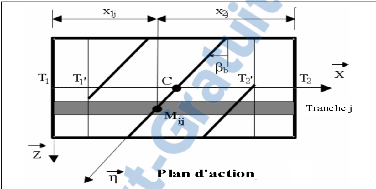
Figure 5.1 : Discretisation des lignes de contact sur le plan d'action.[36]
