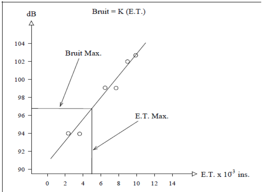
Figure 3.1 : Relation entre l'erreur de transmission et le bruit d'engrènement. (Tho) [15]
