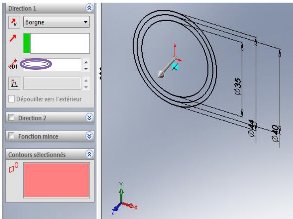
Figure 4.6 : Détermination de la valeur de bossage (extrusion).
