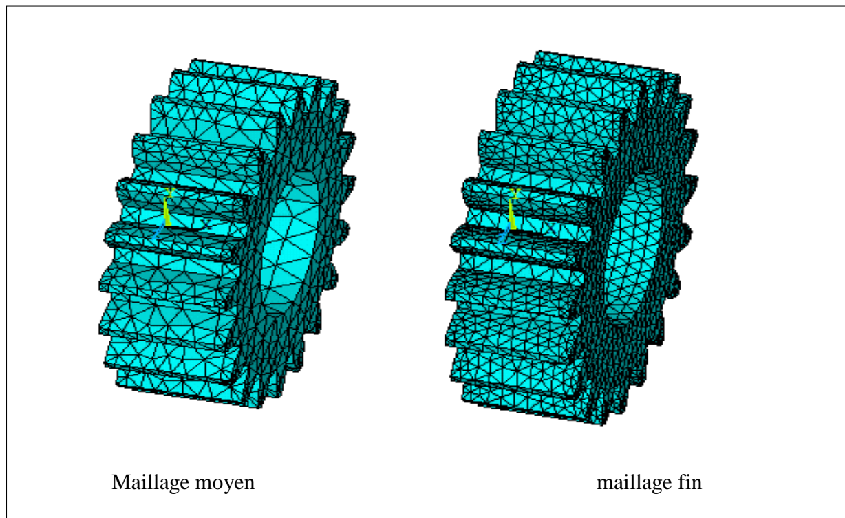
Figure 5.4 : Maillage d'un engrenage à dentures droites.
