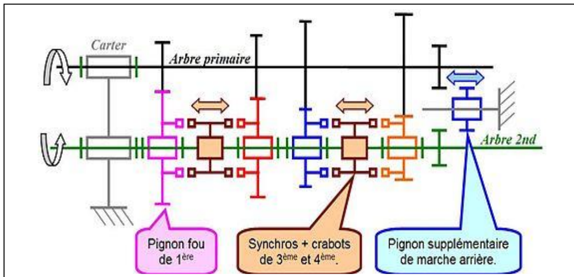
Figure 1.5 : Schéma cinématique du principe d'une boîte de vitesses à 4 rapports et marche arrière. [3]
