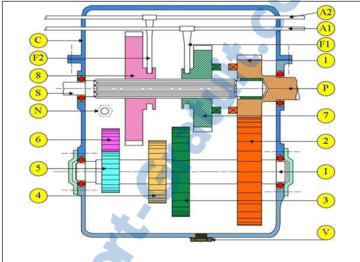
Figure 1.3 : Schéma des organes de la boîte vitesses mécanique. [2]
