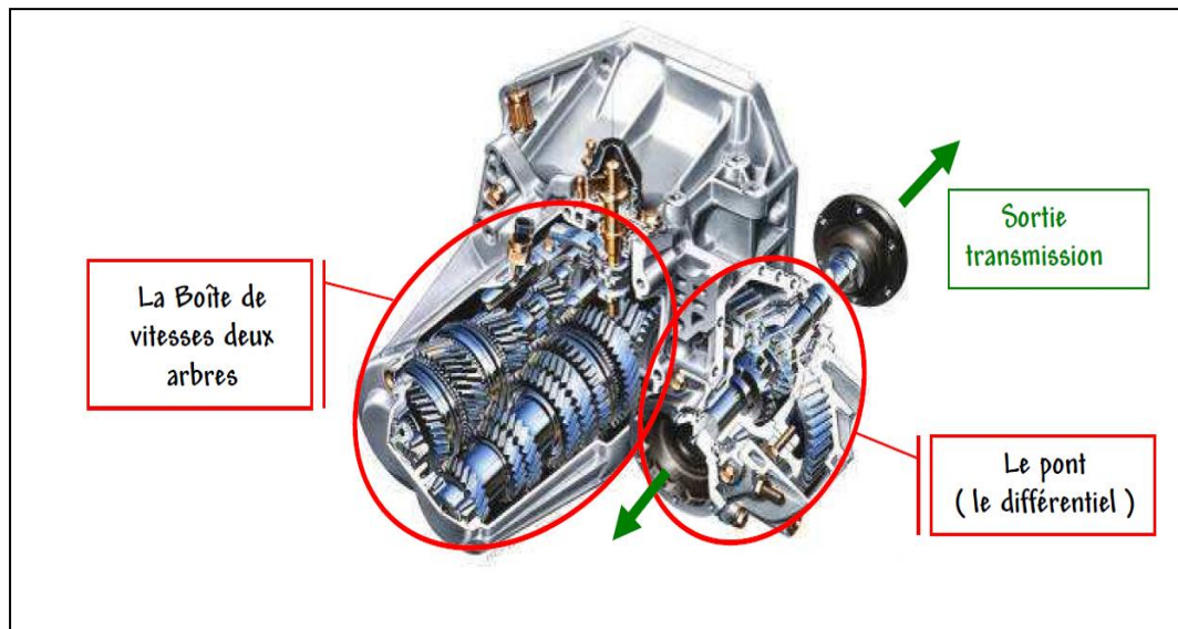
Figure 1.4 : Constitutions de la boîte vitesses. [2]
