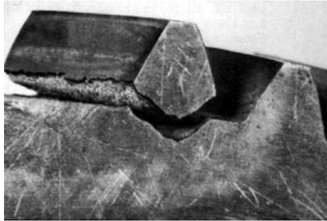
Figure 3.11 : Dent cassée due à aux fissures en pied de dent résultant de la fatigue liée aux charges cycliques de flexion.
