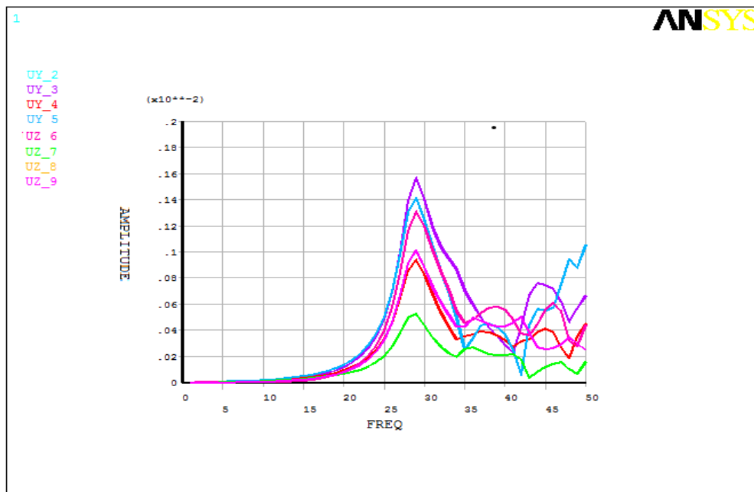
Figure 5.12 : Graphe de la repense fréquentielle cas N° 1(acier).
