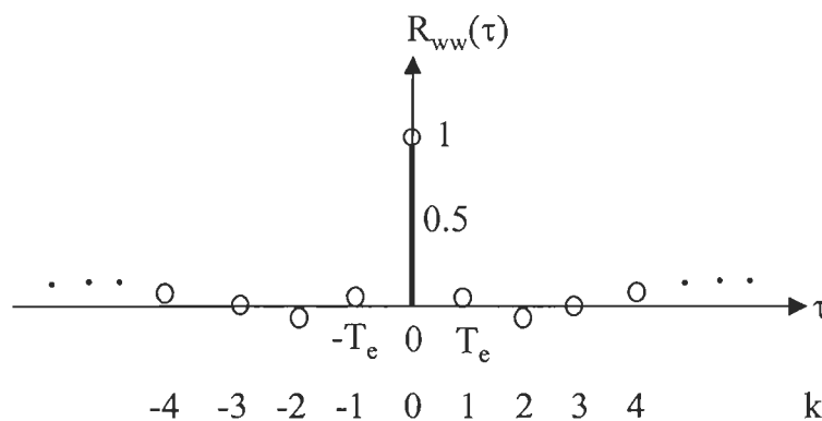
Figure Annexe IX.2 : Représentation des valeurs discrètes de la fonction de corrélation d'un bruit blanc
