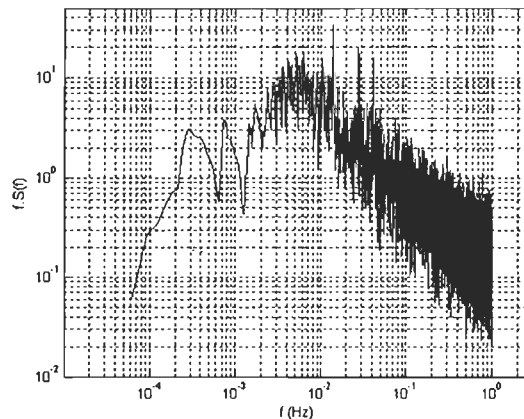
Figure 1.5-39 : Densité spectrale de puissance pour la station Bernatchez
