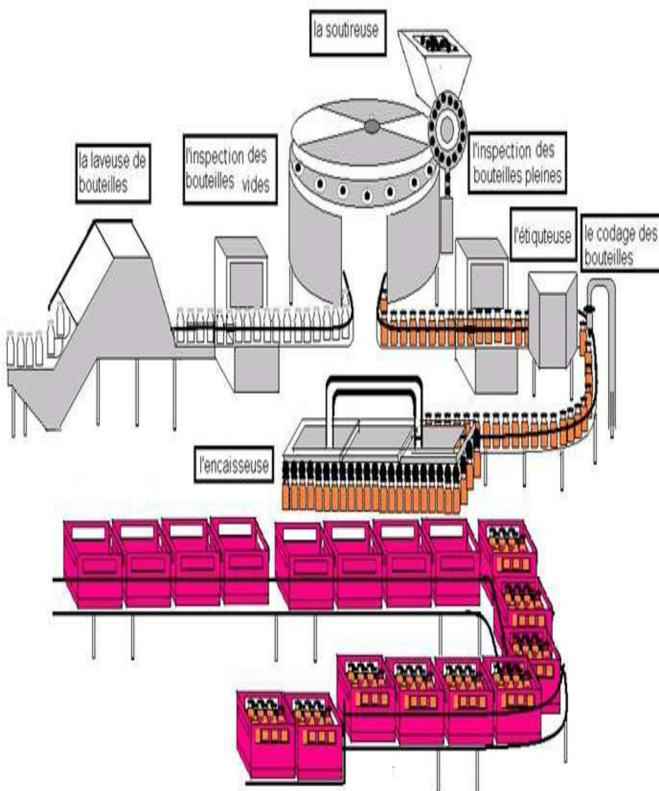
Shémas 1 : les étapes de l'embouteillage des bouteilles en verre
