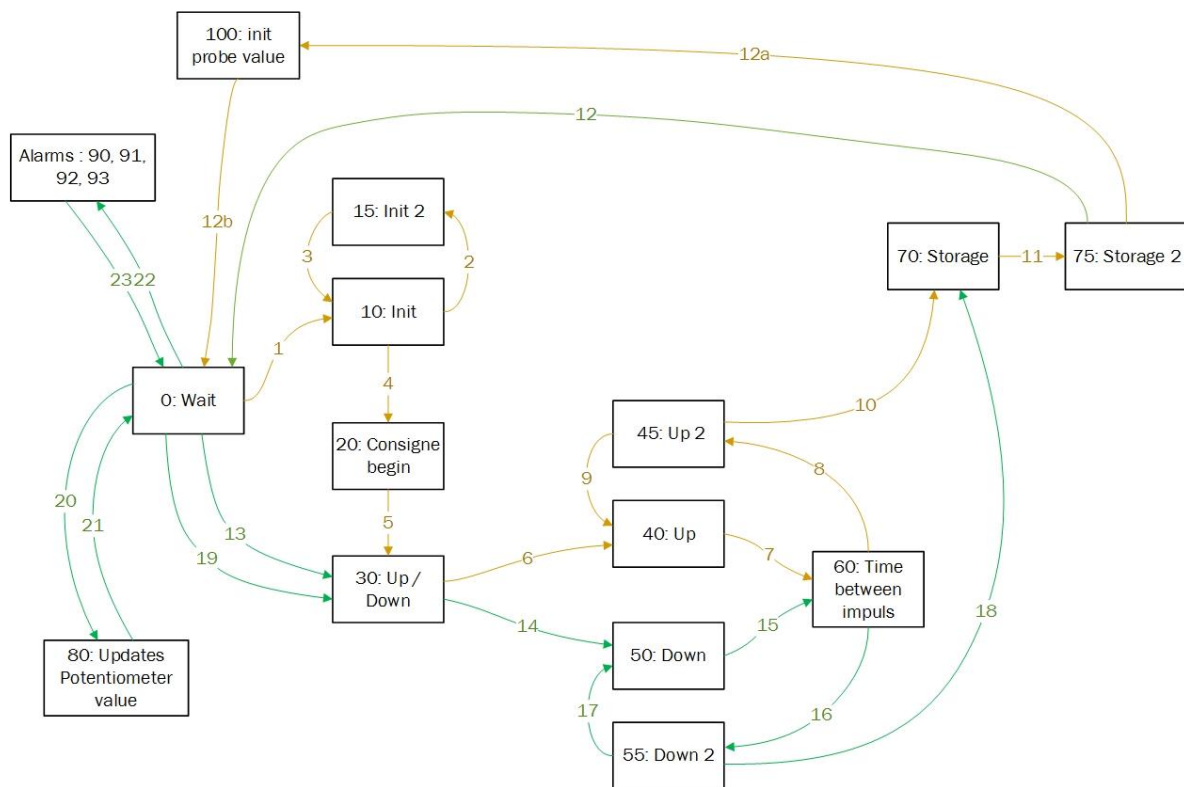
Figure 6 : Machine d'état
