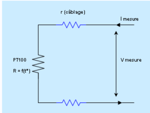
Interface 2 fils
