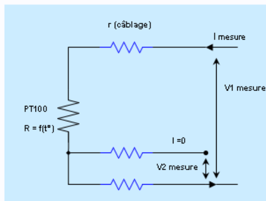
Interface 3 fils
