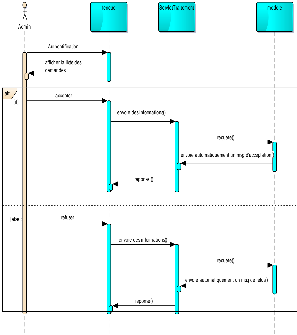
Figure 7 : Diagramme de séquence de traitement des conférences
