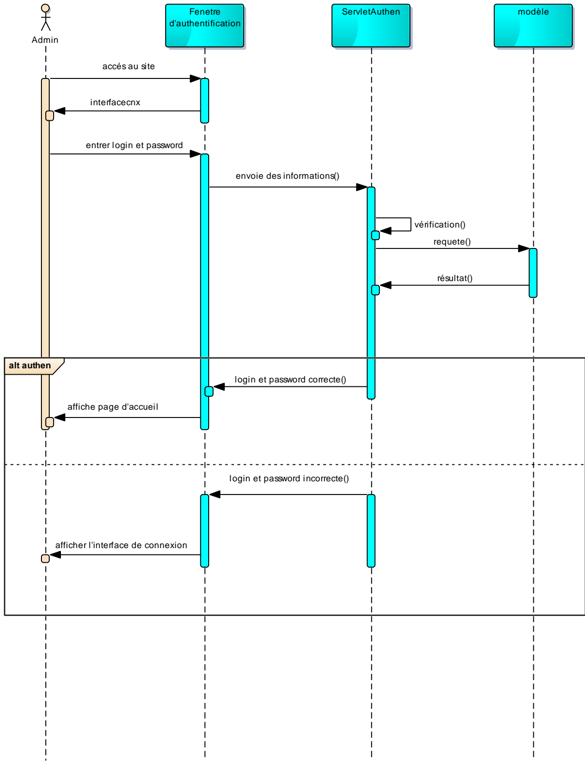
Figure 5 : Diagramme de séquence d'authentification
