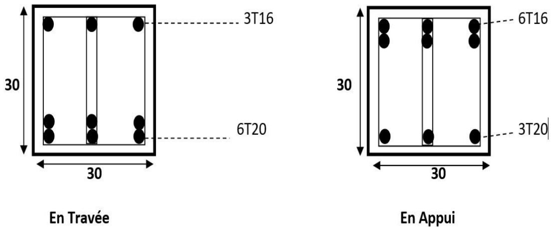
Figure 6.7 Ferrailage des poutres secondaires (30x30) avec f_{c28} = 22 MPa
