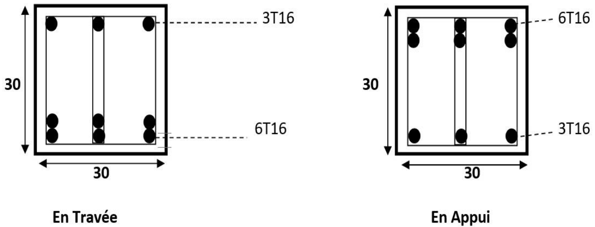
Figure 6.6 Ferrailage des poutres secondaires (30x30) avec f_{c28} = 20 MPa
