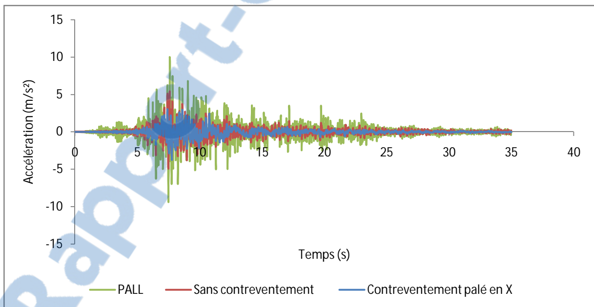
Figure IV.45 : Réponse temporelle de l'accélération.
