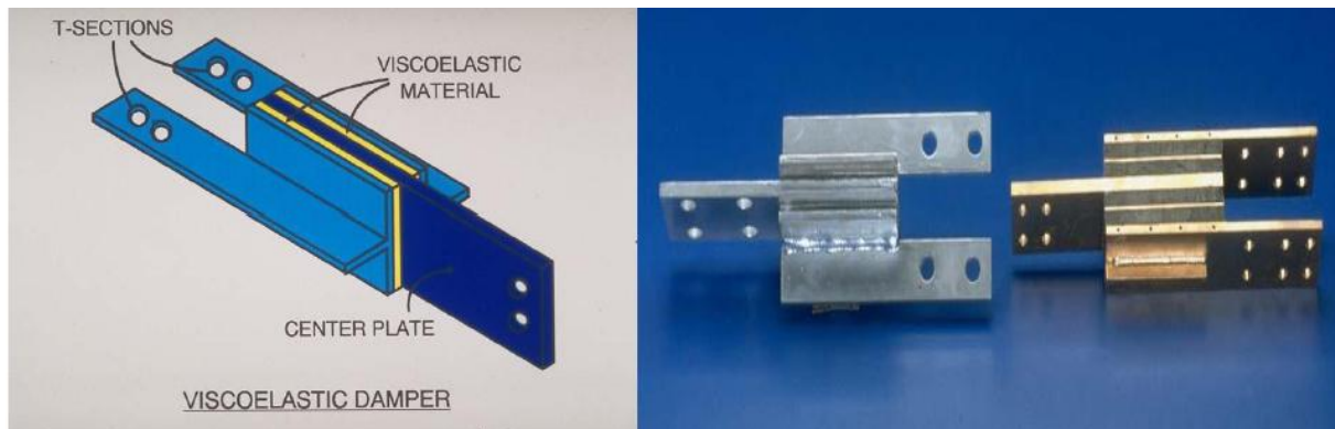
Figure II.9 : Amortisseur visqueux élastique solide [8].
