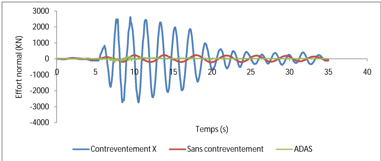
Figure IV.13: Réponse temporelle de l'effort normal.
