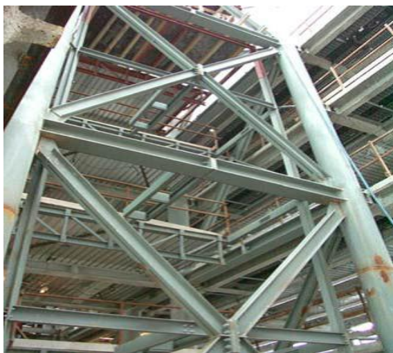
Figure I.7 : Contreventement en diagonales [7].
