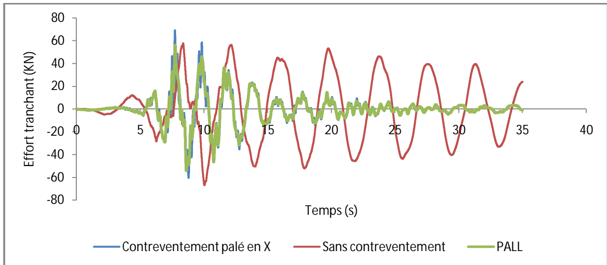
Figure IV.48 : Réponse temporelle de l'effort tranchant.
