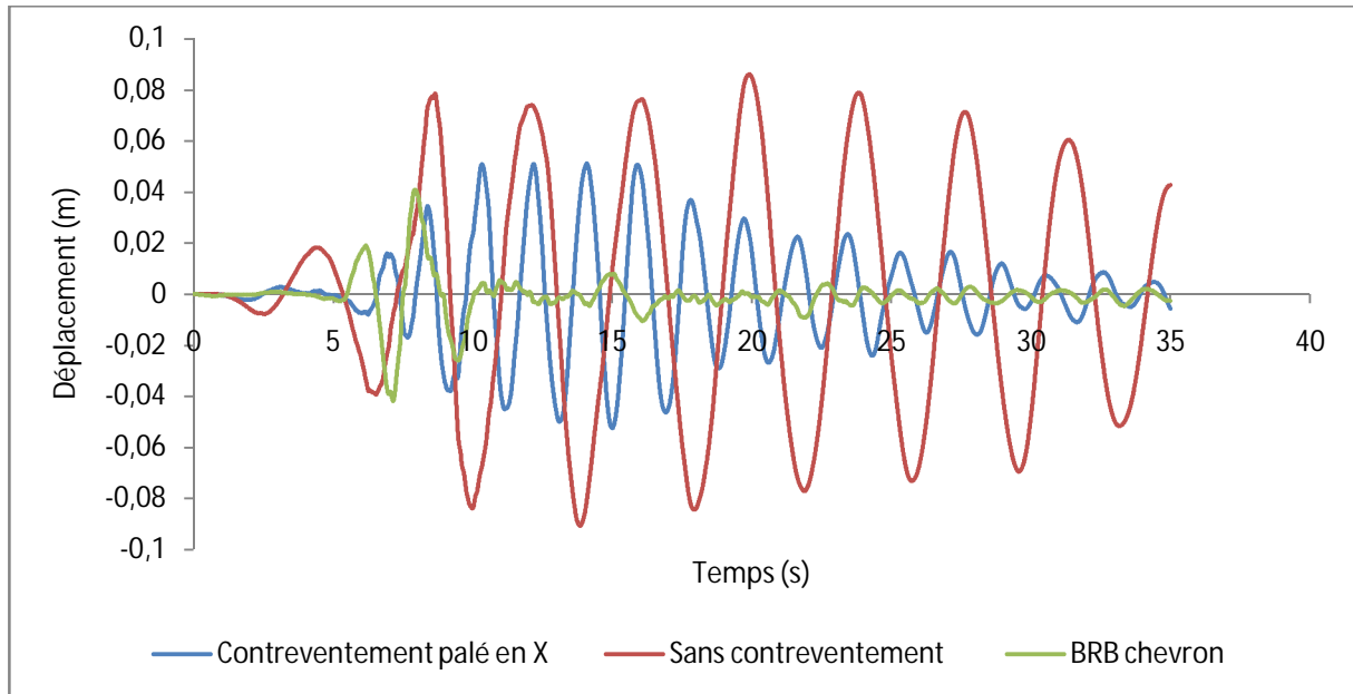
Figure IV.36 : Réponse temporelle du déplacement.
