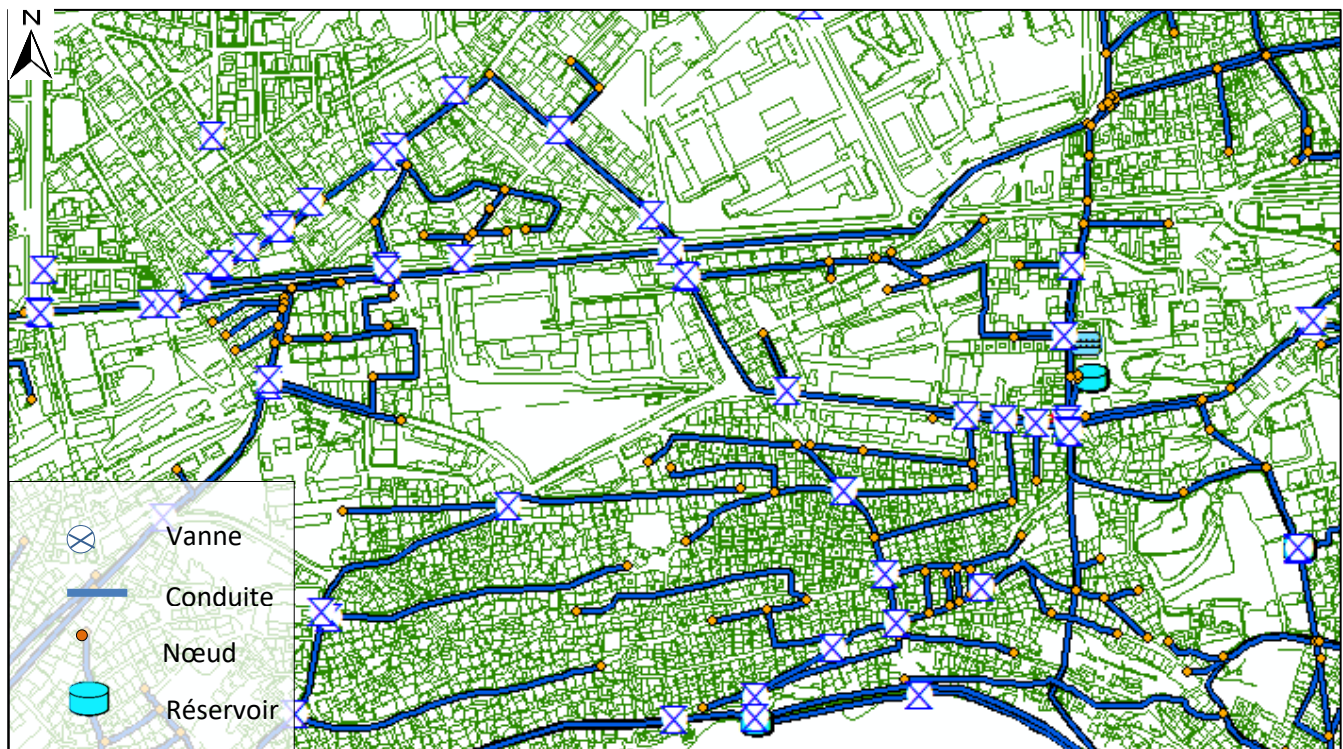
Figure IV.34 : Plan détaillé de la triangulation et de la codification des vannes
