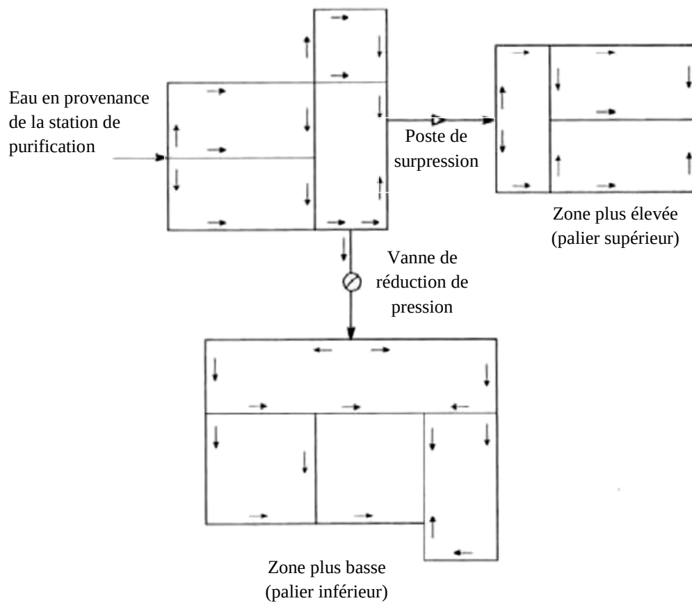
Figure I.8 : Réseaux étagés [3]
