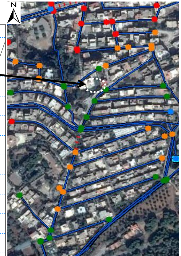
Figure IV.24 : Hauteurs d'eau au nœud 'N202' après modifications
