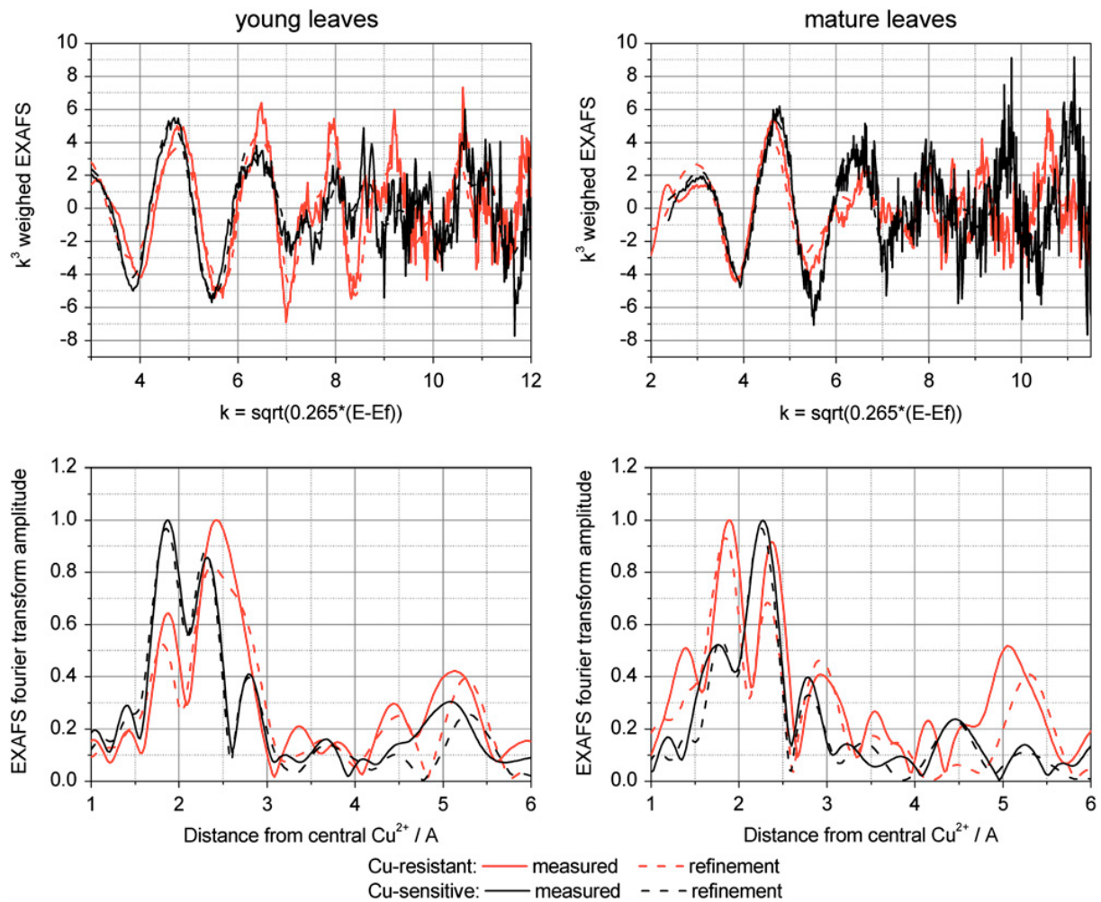
Figure I.8 Spectres EXAFS normalisés et transformées de Fourier des échantillons de feuilles de Thalspi caerulea de l'étude de Mijovilovich et al (2009). Les données sont représentées en traits pleins et les fits en pointillés.
