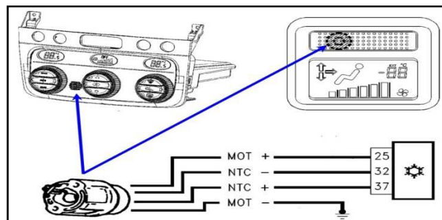
Figure III.5 : capteur de l'air [4]
