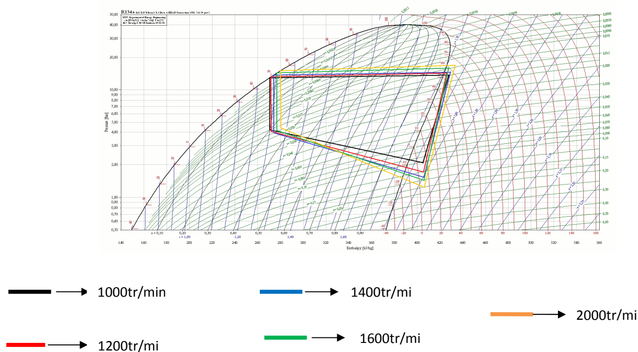
Figure. IV.10. : Diagramme de 2eme étage de ventilation
