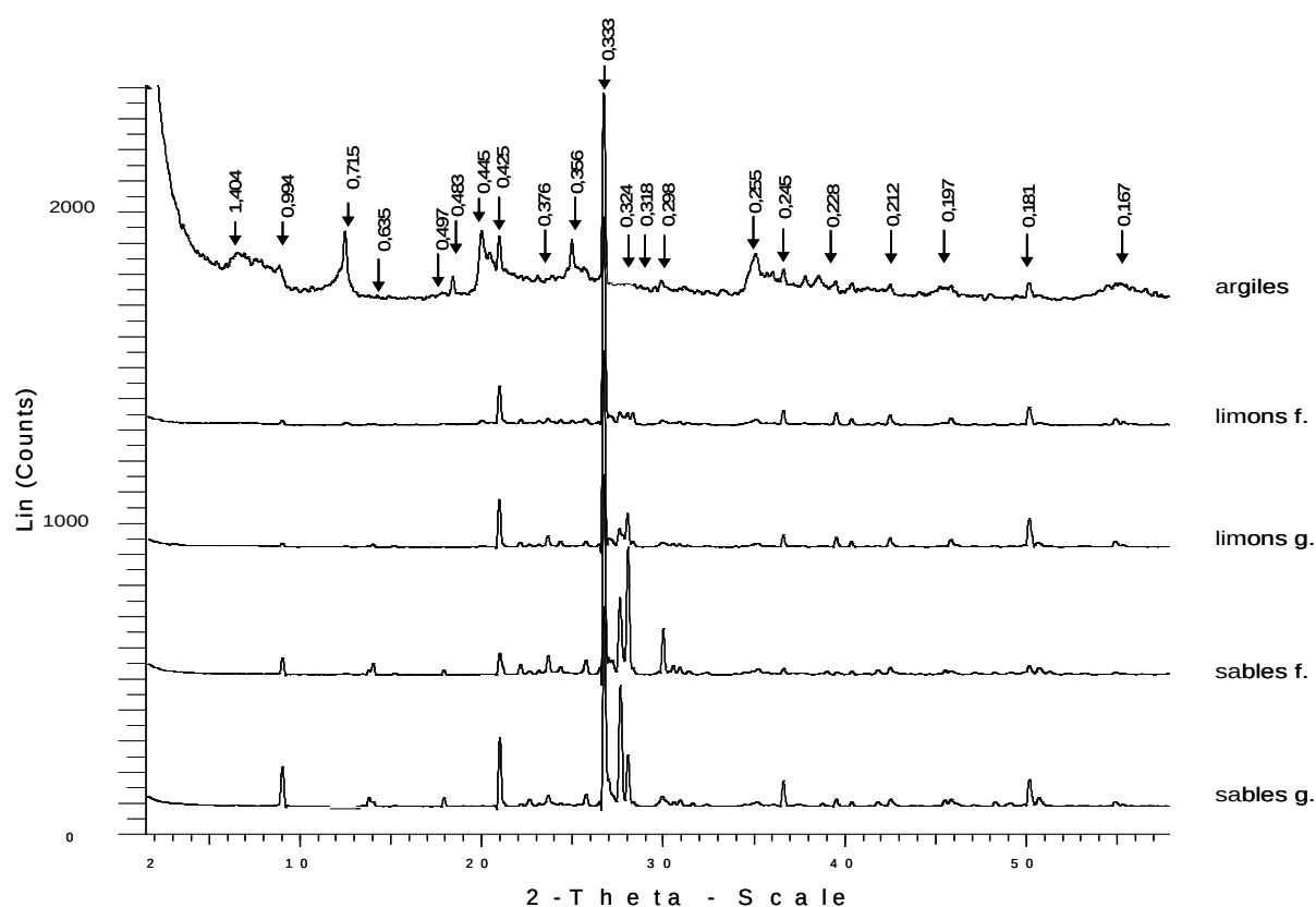
Figure IV.18 : Diffractogrammes des fractions granulométriques de la terre fine acquis sur poudres à 0-5 cm de profondeur.
