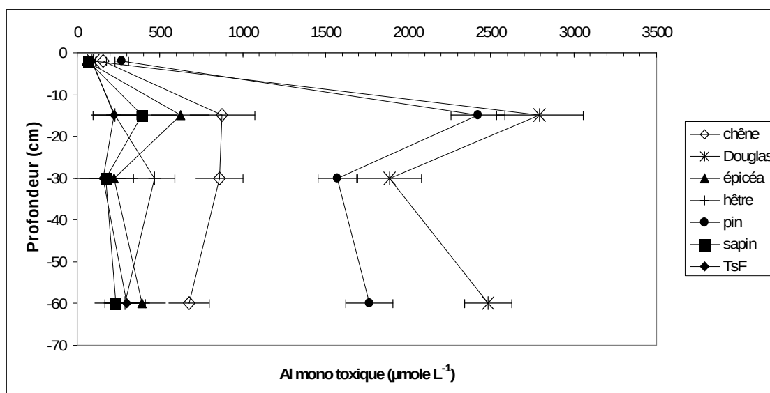
Figure XIX.10 : Concentrations en Al toxique dans les solutions de sol des différents peuplements.
