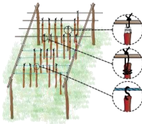
Figure 1 : Schéma du séchoir et des systèmes d'accrochage préconisés par la FAO (FAO, 1990)
