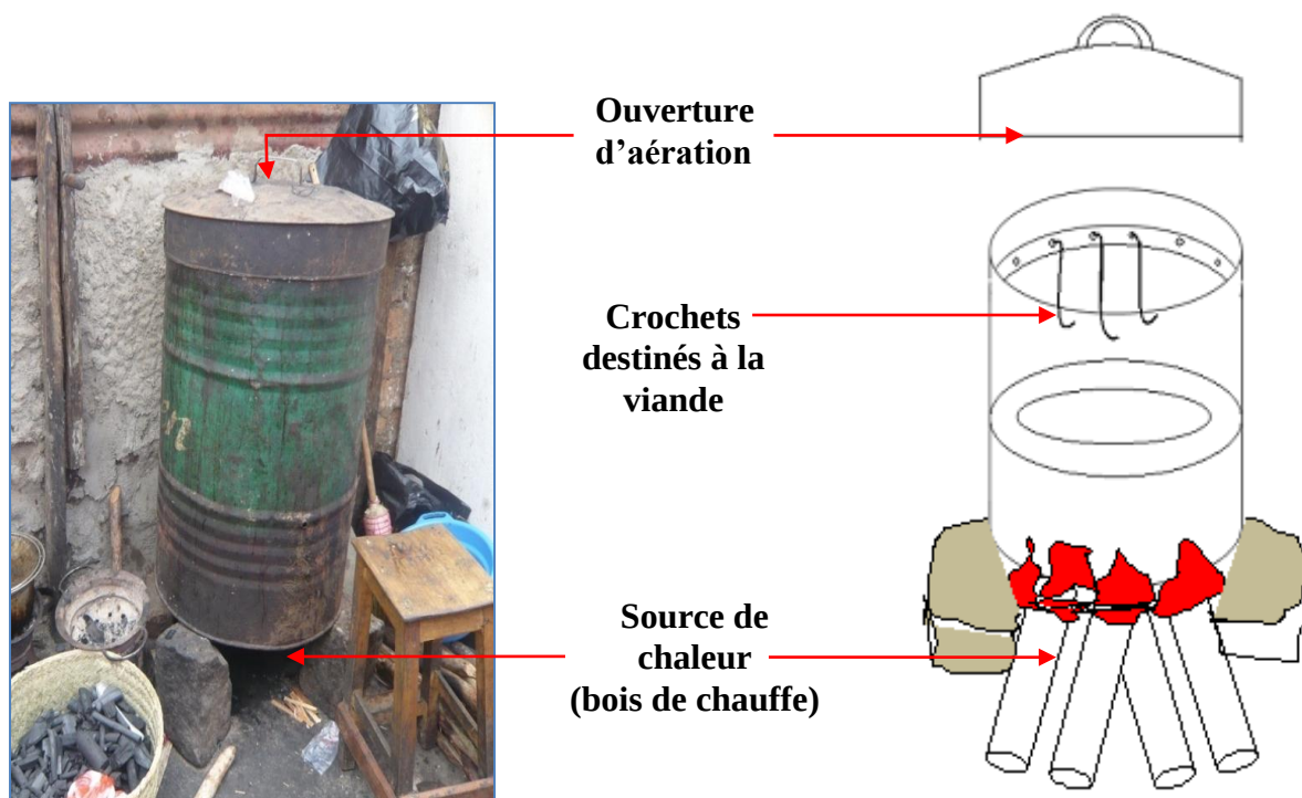
Figure 3b : Modèle de fumoir en tôle
