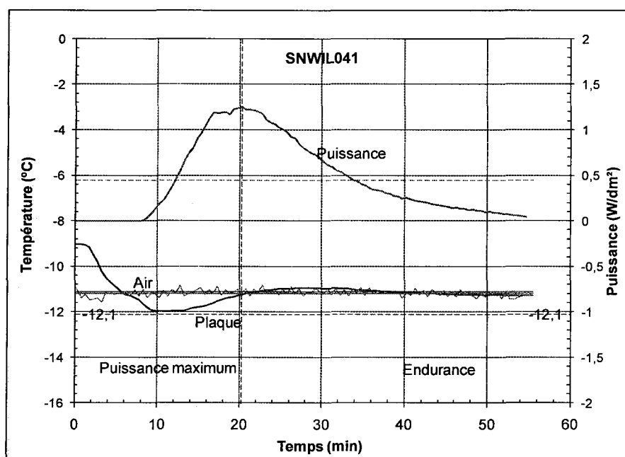
Figure A-17 : Évolution de la puissance et de la température au cours d'un essai de la condition 6 avec une boîte à neige à petits trous, essai SNWIL041
