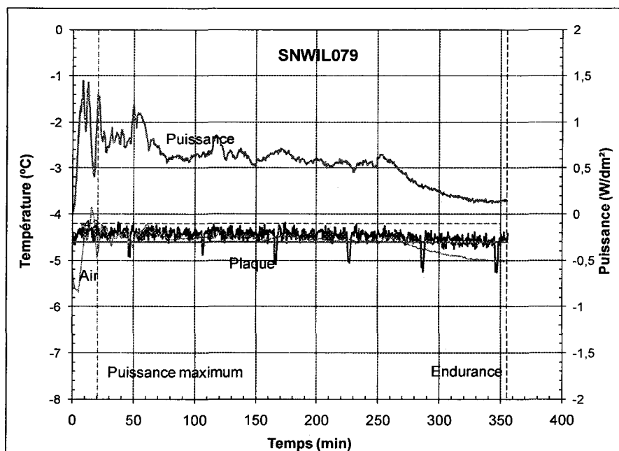
Figure A-1 : Évolution de la puissance et de la température au cours d'un essai de la condition 1 avec une boîte à neige à petits trous, essai SNWIL079
