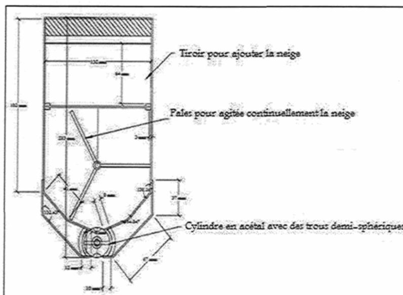
Figure 14 : Coupe transversale de la boîte à neige
