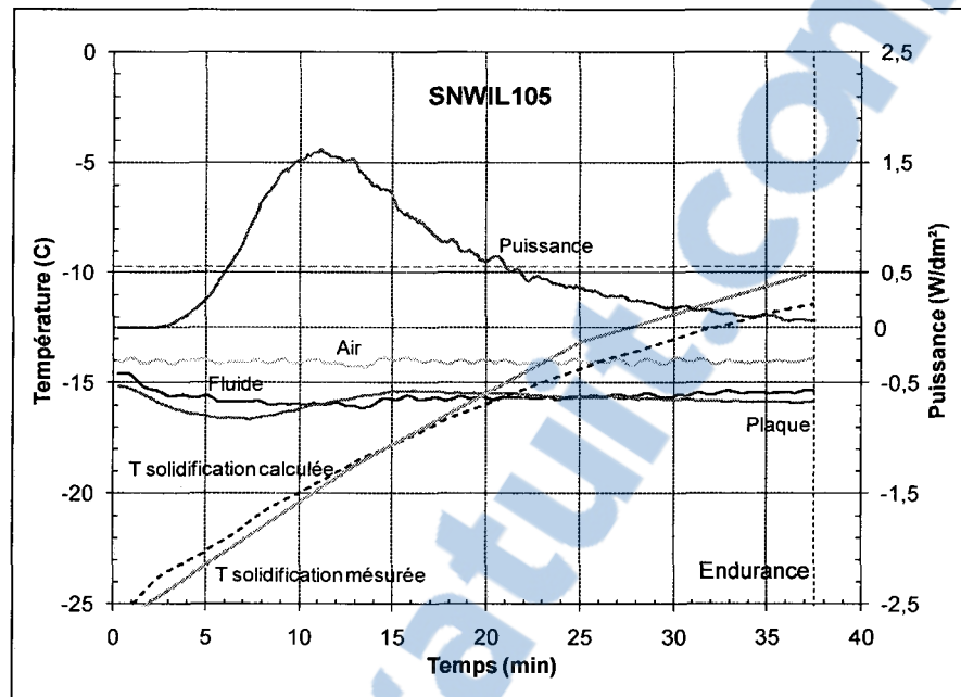
Figure B-7 : Évolution de la puissance et des températures dans le temps pour l'essai SNWIL105
