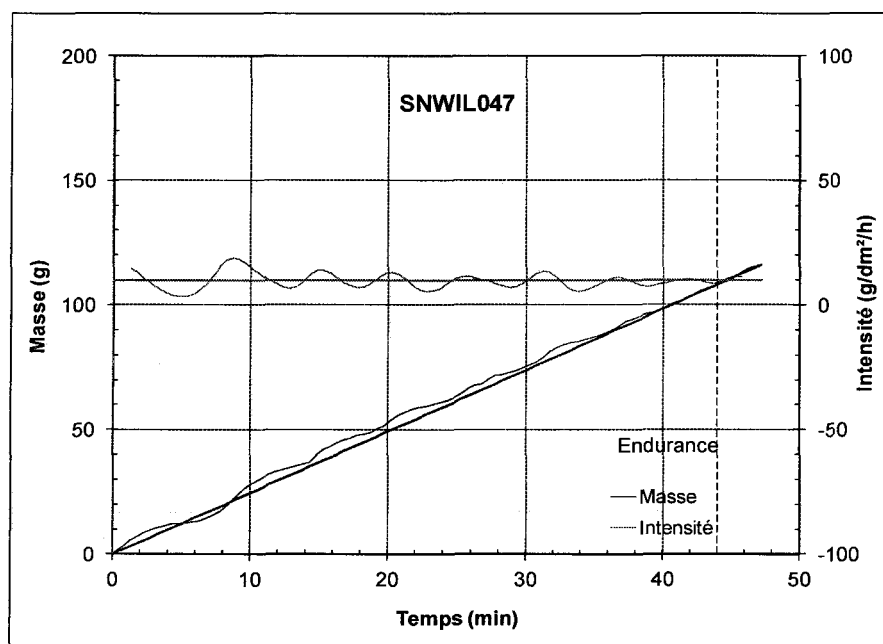
Figure 38 : Évolution de la masse et de l'intensité au cours d'un essai de la condition 4 avec une boîte à neige à petits trous, essai SNWIL047
