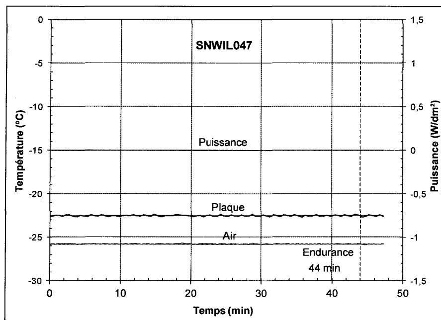
Figure 37 : Évolution de la puissance et de la température au cours d'un essai de la condition 4 avec une boîte à neige à petits trous, essai SNWIL047
