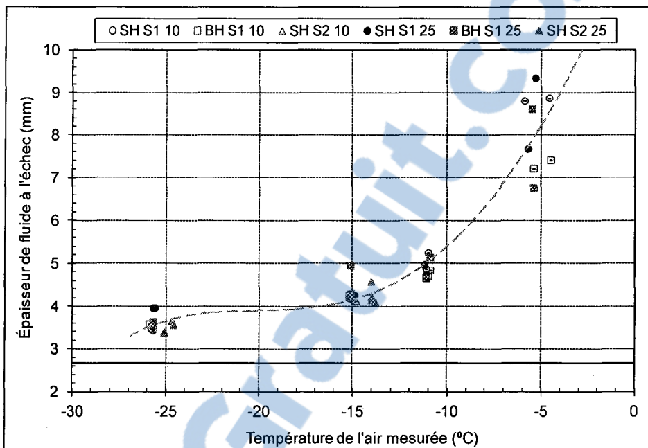
Figure 79 : Épaisseur finale de neige qui tombe sur le fluide
