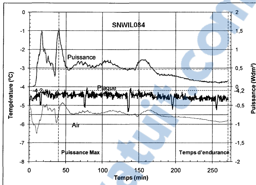
Figure A-3 : Évolution de la puissance et de la température au cours d'un essai de la condition 1 avec une boîte à neige à gros trous, essai SNWIL084
