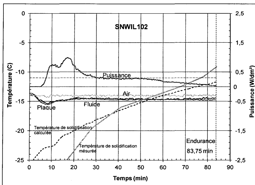
Figure 60 : Évolution de la puissance et des températures dans le temps pour l'essai SNWIL102
