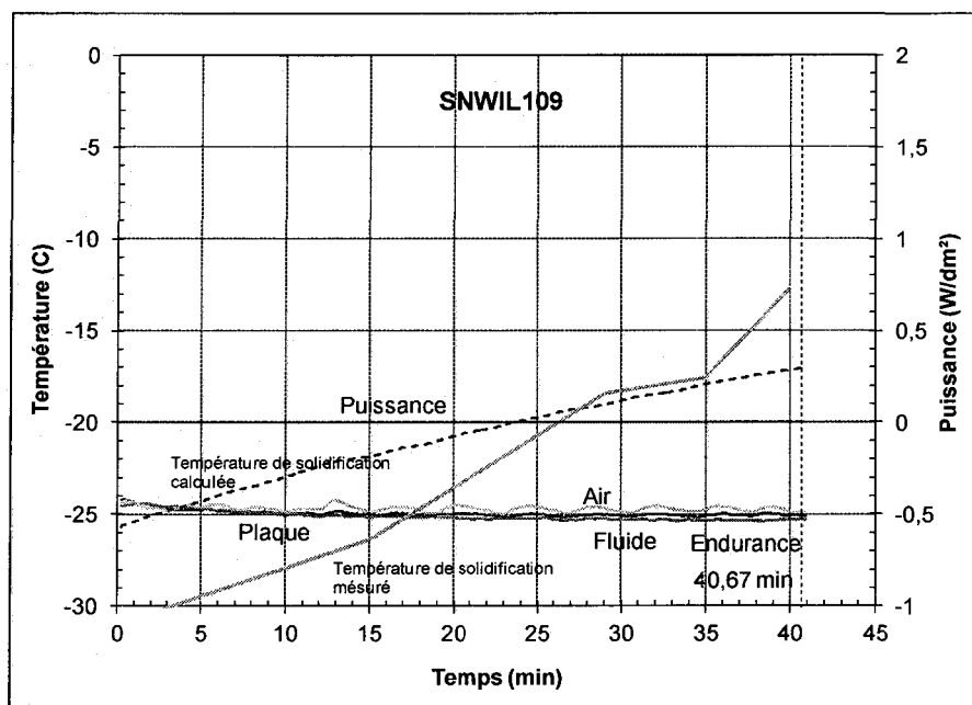
Figure 63 : Évolution de la puissance et des températures dans le temps pour l'essai SNWIL109
