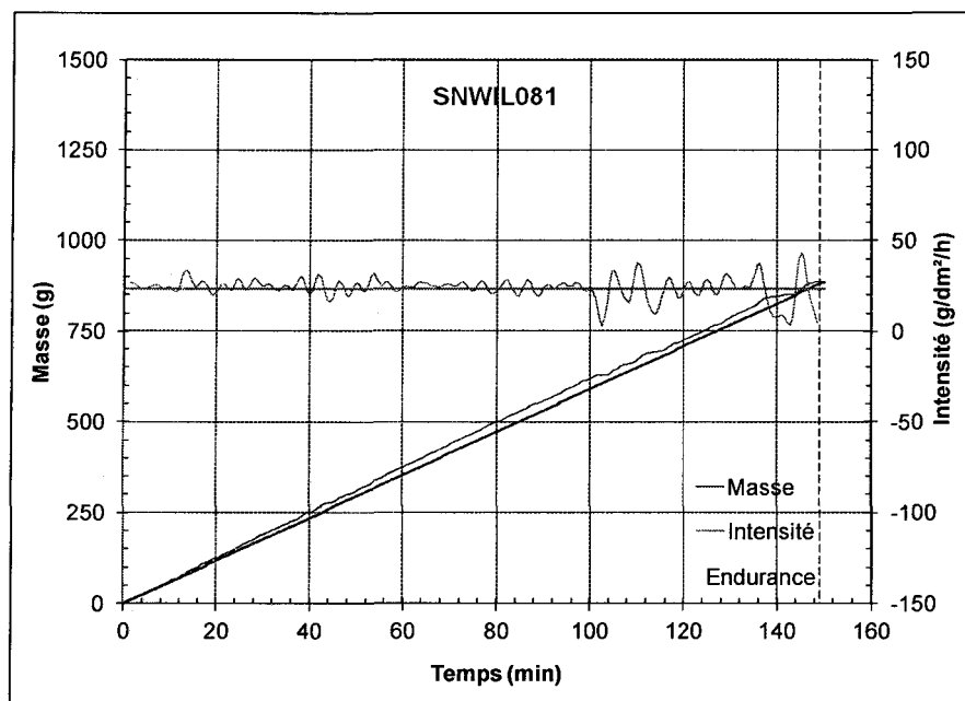
Figure A-16 : Évolution de la masse et de l'intensité des précipitations de neige au cours d'un essai de la condition 5 avec une boîte à neige à gros trous, essai SNWIL081
