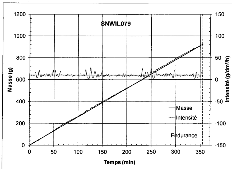
Figure A-2 : Évolution de la masse et de l'intensité des précipitations de neige au cours d'un essai de la condition 1 avec une boîte à neige à petits trous, essai SNWIL079
