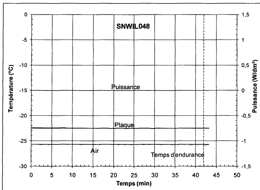
Figure A-9 : Évolution de la puissance et de la température au cours d'un essai de la condition 4 avec une boîte à neige à petits trous, essai SNWIL048
