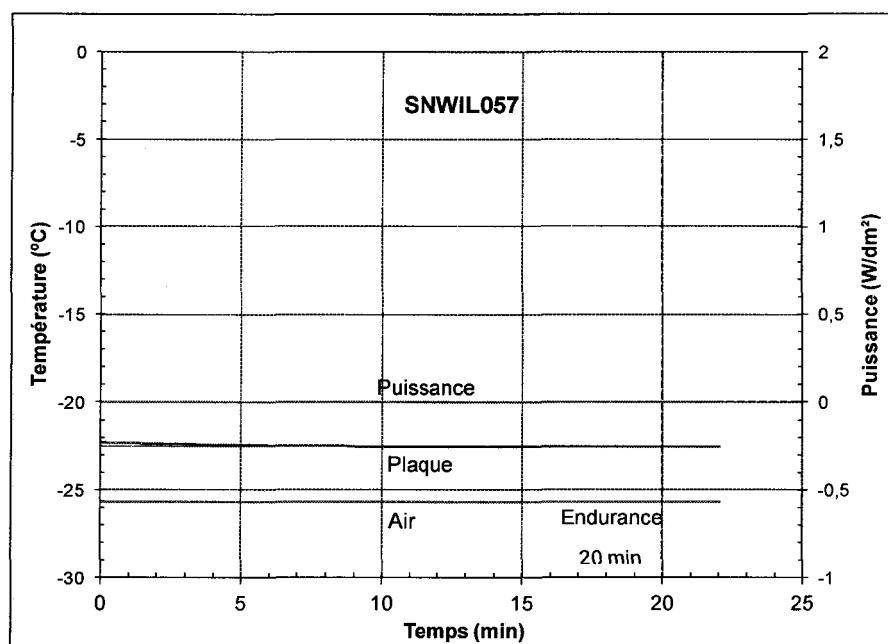
Figure 55 : Évolution de la puissance et de la température au cours d'un essai de la condition 8 avec une boîte à neige à gros trous, essai SNWIL057
