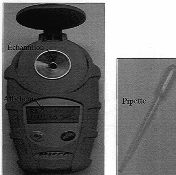
Figure 19 : Réfractomètre numérique MISCO Palm Abbe N°: PA-202X
