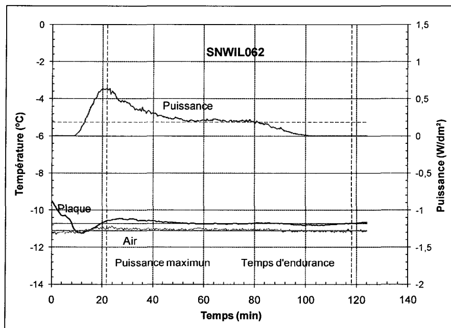
Figure A-5 : Évolution de la puissance et de la température au cours d'un essai de la condition 2 avec une boîte à neige à petits trous, essai SNWIL062
