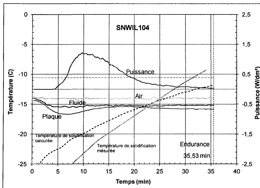
Figure 69 : Évolution de la puissance et des températures dans le temps pour l'essai SNWIL104
