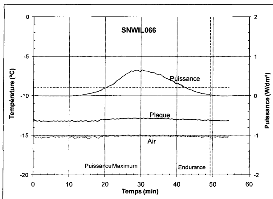
Figure A-23 : Évolution de la puissance et de la température au cours d'un essai de la condition 7 avec une boîte à neige à gros trous, essai SNWIL066
