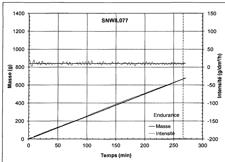
Figure 28 : Évolution de la masse et de l'intensité au cours d'un essai de la condition 1 avec une boîte à neige à gros trous, essai SNWIL077
