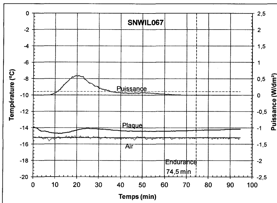
Figure 35 : Évolution de la puissance et de la température au cours d'un essai de la condition 3 avec une boîte à neige à gros trous, essai SNWIL067
