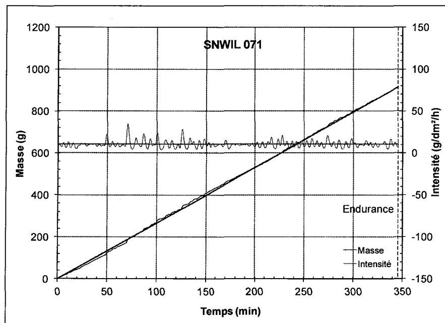
Figure 26 : Évolution de la masse et de l'intensité au cours d'un essai de la condition 1 avec une boîte à neige à petits trous, essai SNWIL071
