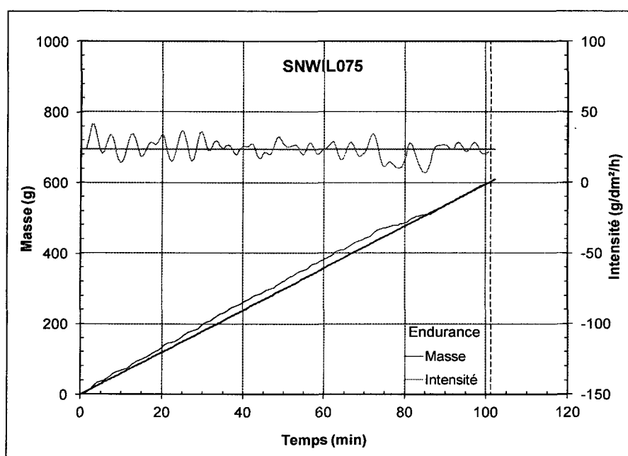
Figure 44 : Évolution de la masse et de l'intensité au cours d'un essai de la condition 5 avec une boîte à neige à gros trous, essai SNWIL075
