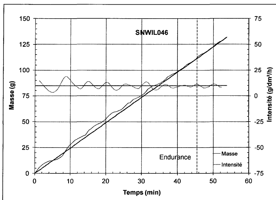
Figure A-12 : Évolution de la masse et de l'intensité des précipitations de neige au cours d'un essai de la condition 4 avec une boîte à neige à gros trous, essai SNWIL046
