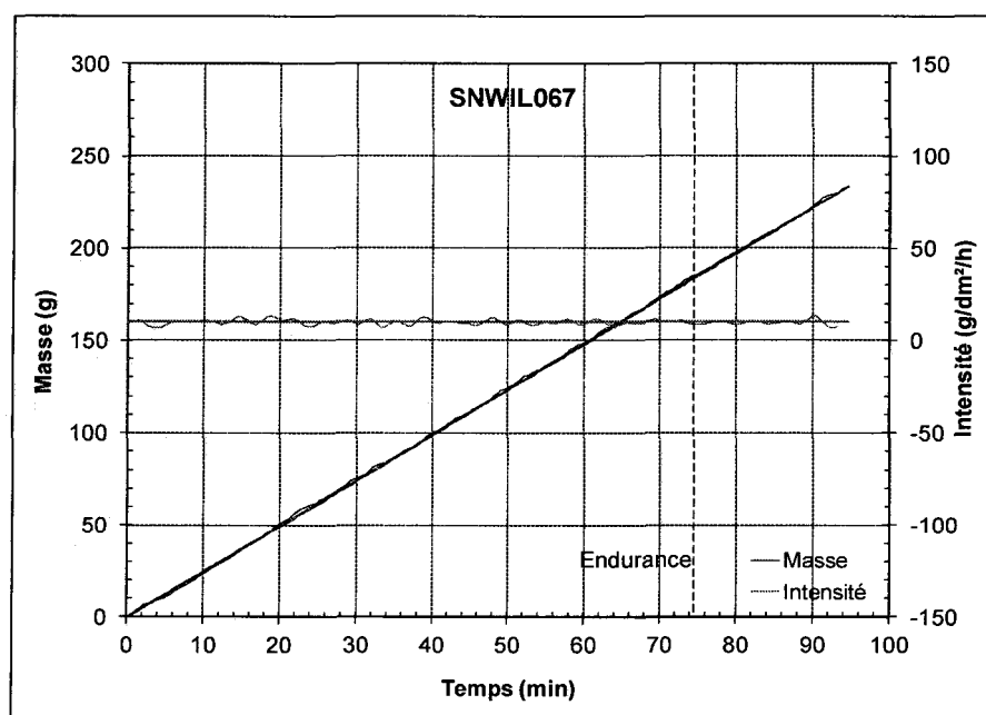
Figure 36 : Évolution de la masse et de l'intensité au cours d'un essai de la condition 3 avec une boîte à neige à petits trous, essai SNWIL067
