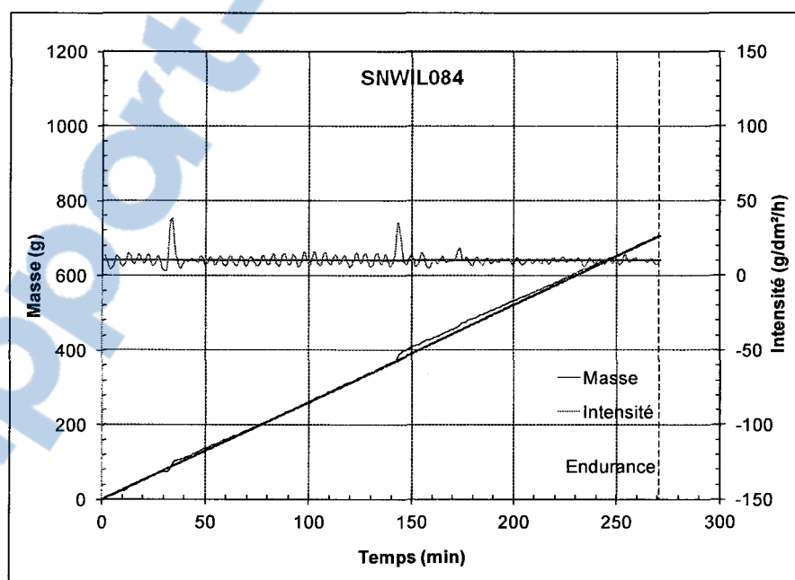
Figure A-4 : Évolution de la masse et de l'intensité des précipitations de neige au cours d'un essai de la condition 1 avec une boîte à neige à gros trous, essai SNWIL084
