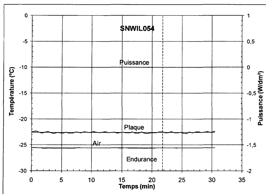
Figure A-25 : Évolution de la puissance et de la température au cours d'un essai de la condition 8 avec une boîte à neige à petits trous, essai SNWIL054
