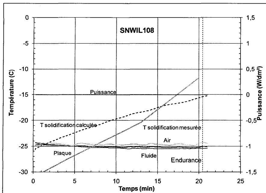
Figure B-11 : Évolution de la puissance et des températures dans le temps pour l'essai SNWIL108
