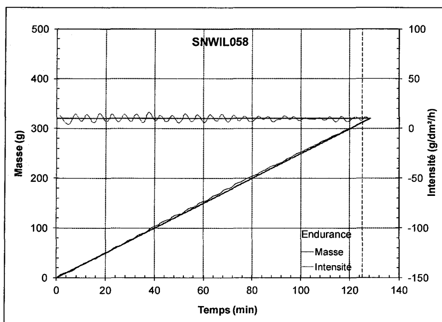
Figure 32 : Évolution de la masse et de l'intensité au cours d'un essai de la condition 2 avec une boîte à neige à gros trous, essai SNWIL058
