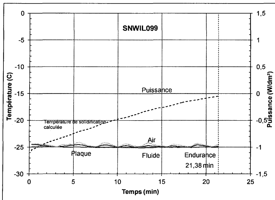
Figure 71 : Évolution de la puissance et des températures dans le temps pour l'essai SNWIL099
