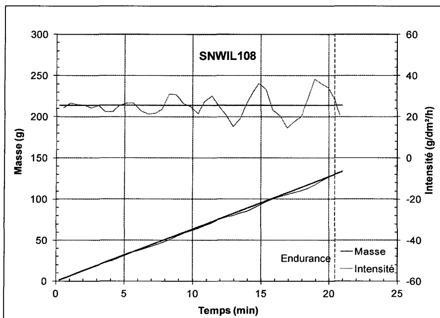
Figure B-12 : Évolution de l'intensité et de la masse des précipitations de neige dans le temps pour l'essai SNWIL108
