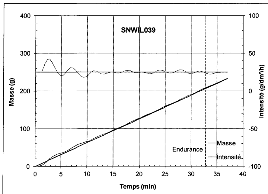
Figure A-22 : Évolution de la masse et de l'intensité des précipitations de neige au cours d'un essai de la condition 7 avec une boîte à neige à petits trous, essai SNWIL039
