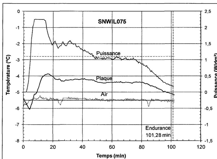
Figure 43 : Évolution de la puissance et de la température au cours d'un essai de la condition 5 avec une boîte à neige à gros trous, essai SNWIL075
