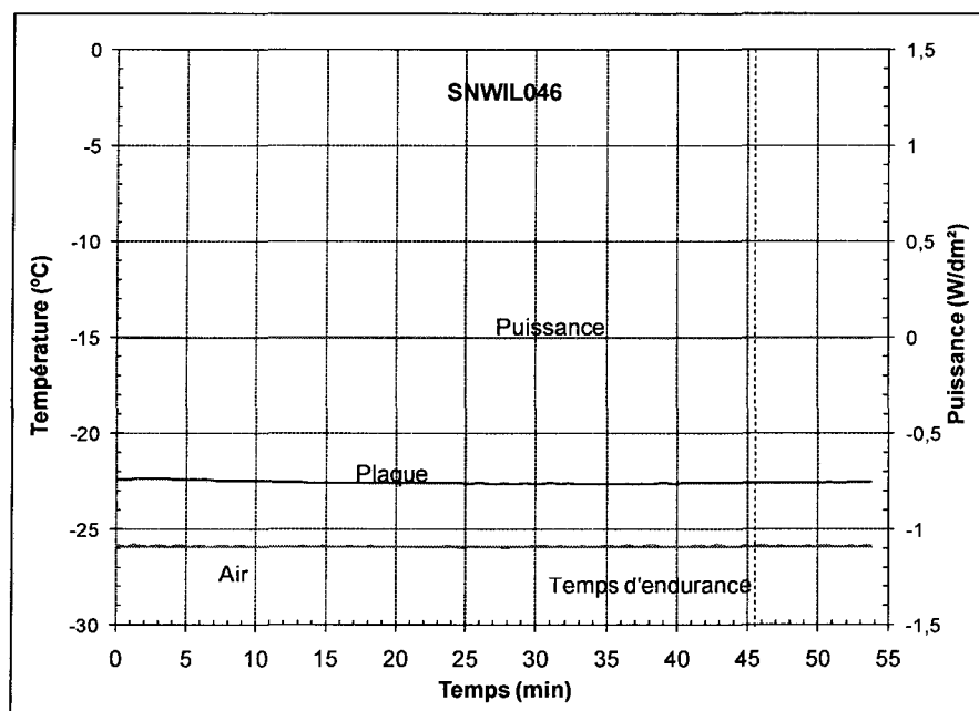
Figure A-11 : Évolution de la puissance et de la température au cours d'un essai de la condition 4 avec une boîte à neige à gros trous, essai SNWIL046
