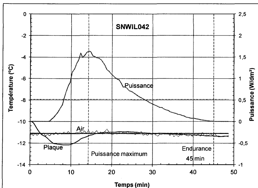
Figure 45 : Évolution de la puissance et de la température au cours d'un essai de la condition 6 avec une boîte à neige à petits trous, essai SNWIL042
