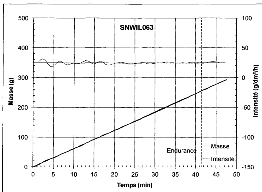
Figure A-20 : Évolution de la masse et de l'intensité des précipitations de neige au cours d'un essai de la condition 6 avec une boîte à neige à gros trous, essai SNWIL063
