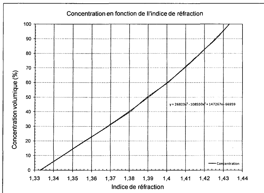
Figure 20 : Concentration de propylène glycol en fonction de l'indice de réfraction
