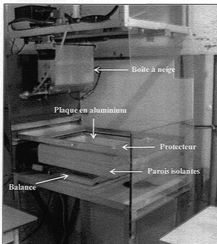
Figure 13 : Système de distribution de neige
