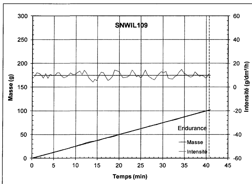
Figure 64 : Évolution de l'intensité des précipitations et de la masse de neige dans le temps pour l'essai SNWIL109
