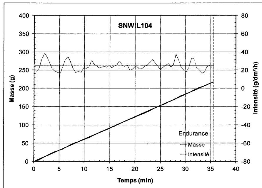
Figure 70 : Évolution de l'intensité des précipitations et de la masse de neige dans le temps pour l'essai SNWIL104
