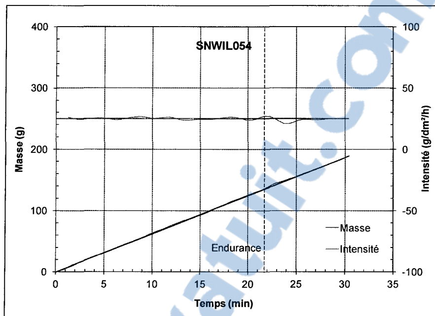
Figure A-26 : Évolution de la masse et de l'intensité des précipitations de neige au cours d'un essai de la condition 8 avec une boîte à neige à petits trous, essai SNWIL054
