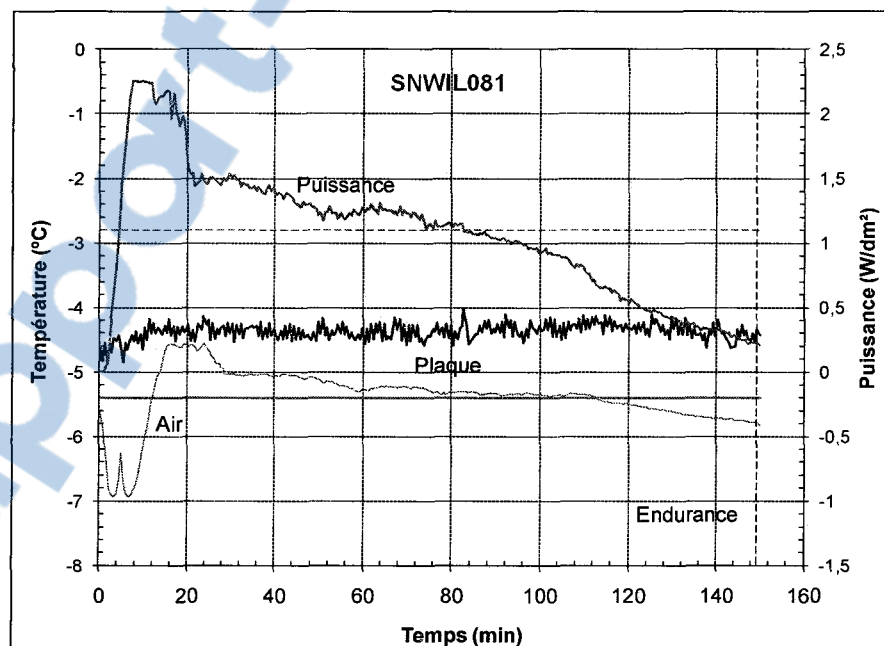
Figure A-15 : Évolution de la puissance et de la température au cours d'un essai de la condition 5 avec une boîte à neige à gros trous, essai SNWIL081
