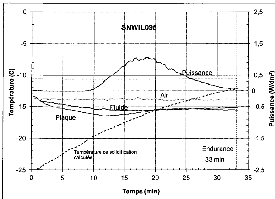
Figure 67 : Évolution de la puissance et des températures dans le temps pour l'essai SNWIL095
