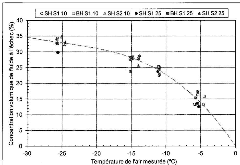
Figure 80 : Concentration finale en propylène glycol dans le fluide
