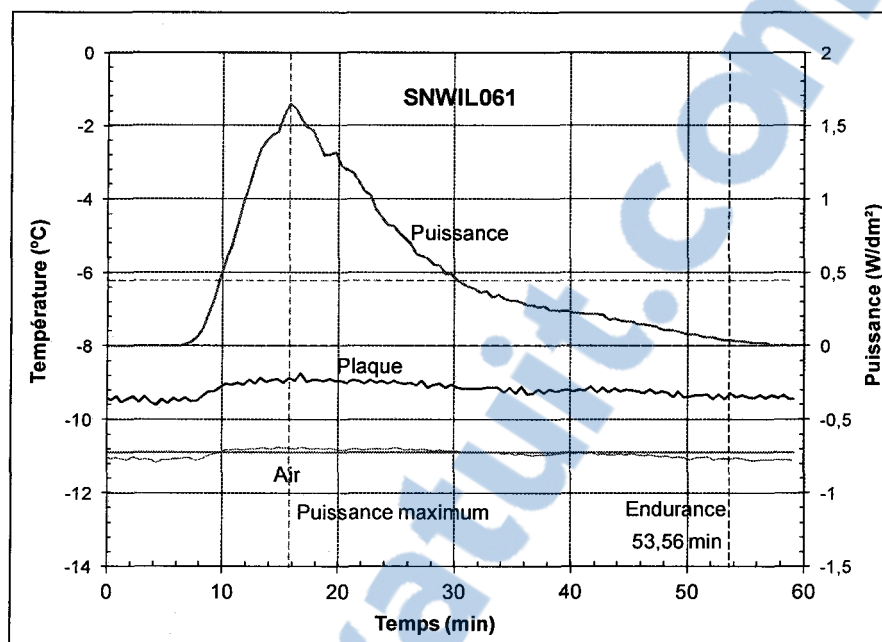
Figure 47 : Évolution de la puissance et de la température au cours d'un essai de la condition 6 avec une boîte à neige à gros trous, essai SNWIL061
