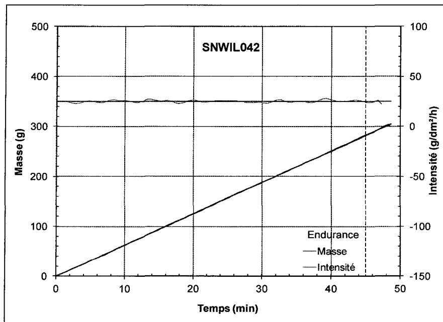
Figure 46 : Évolution de la masse et de l'intensité au cours d'un essai de la condition 6 avec une boîte à neige à petits trous, essai SNWIL042
