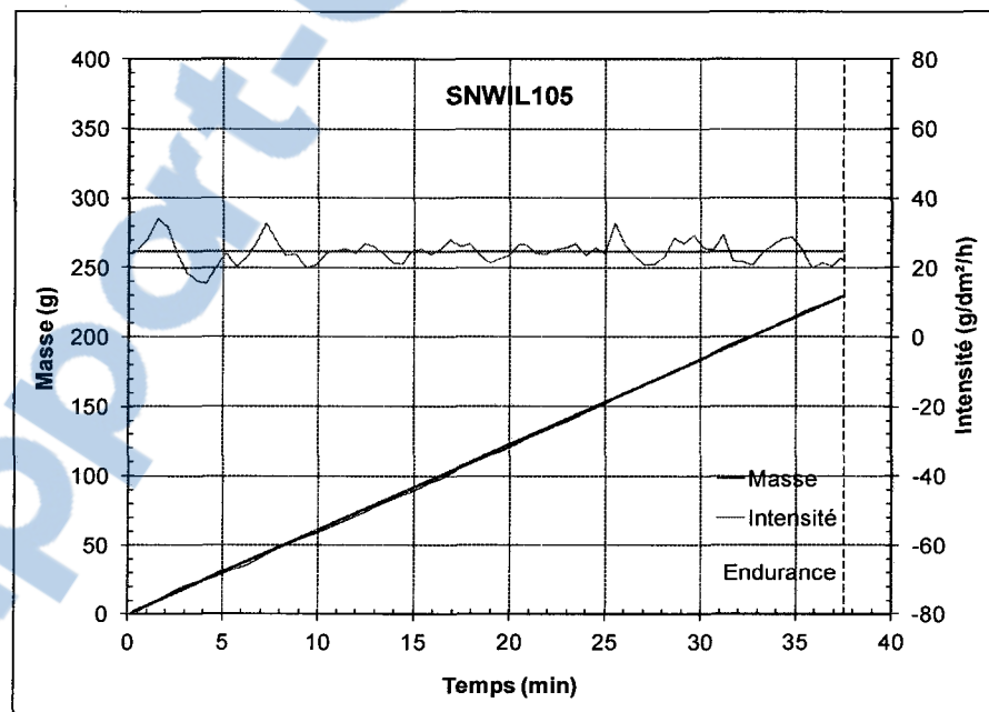
Figure B-8 : Évolution de l'intensité et de la masse des précipitations de neige dans le temps pour l'essai SNWIL105
