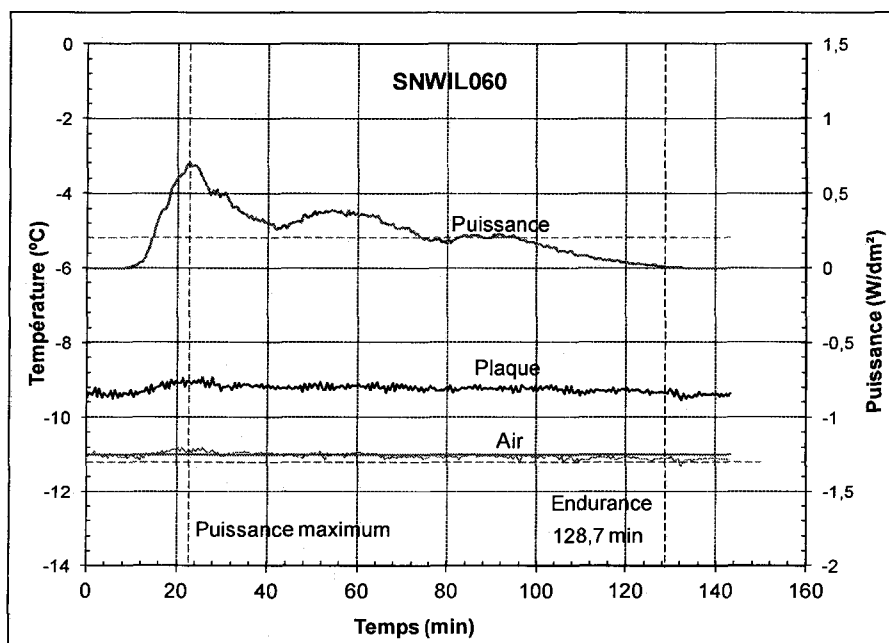
Figure 29 : Évolution de la puissance et de la température au cours d'un essai de la condition 2 avec une boîte à neige à petits trous, essai SNWIL060
