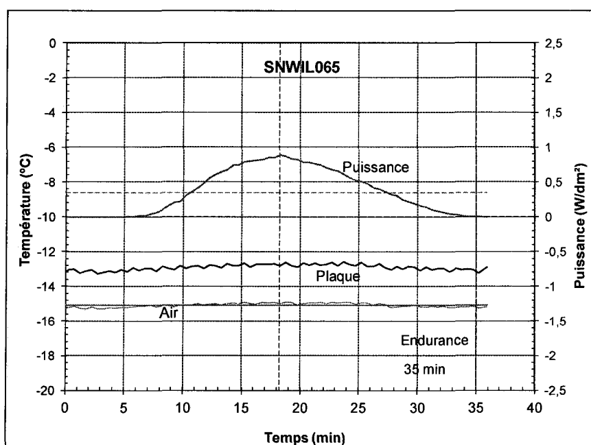
Figure 49 : Évolution de la puissance et de la température au cours d'un essai de la condition 7 avec une boîte à neige à petits trous, essai SNWIL065
