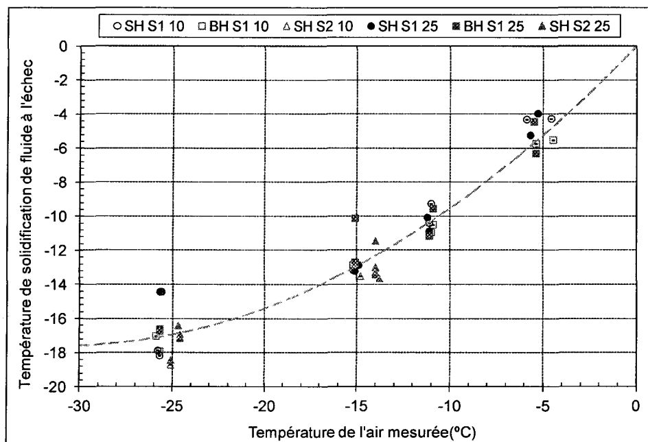
Figure 83 : Température de solidification finale du fluide
