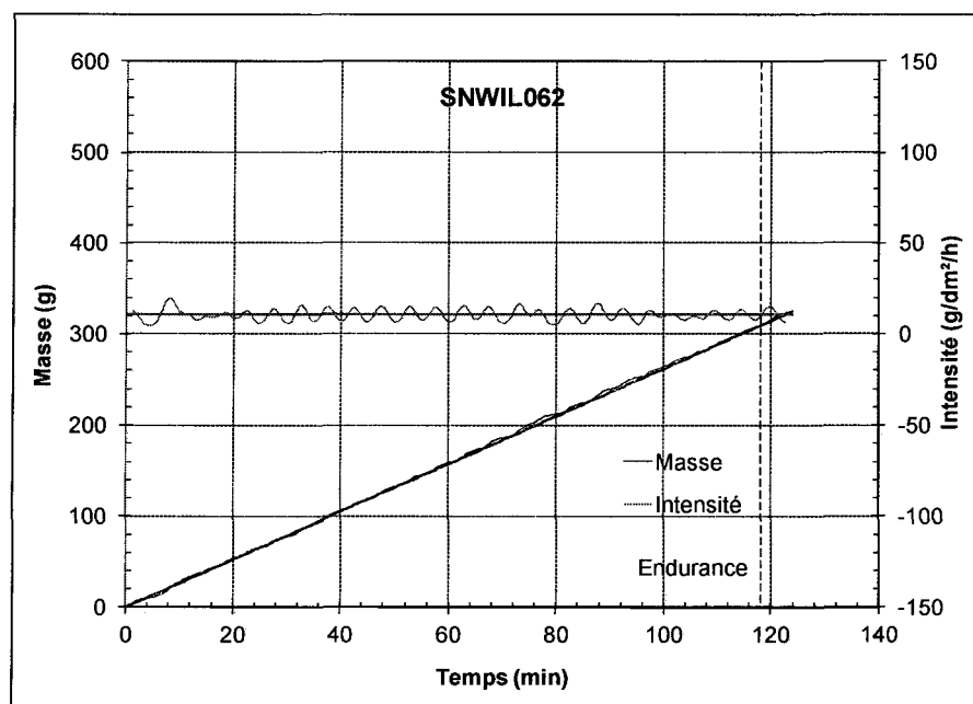
Figure A-6 : Évolution de la masse et de l'intensité des précipitations de neige au cours d'un essai de la condition 2 avec une boîte à neige à petits trous, essai SNWIL062
