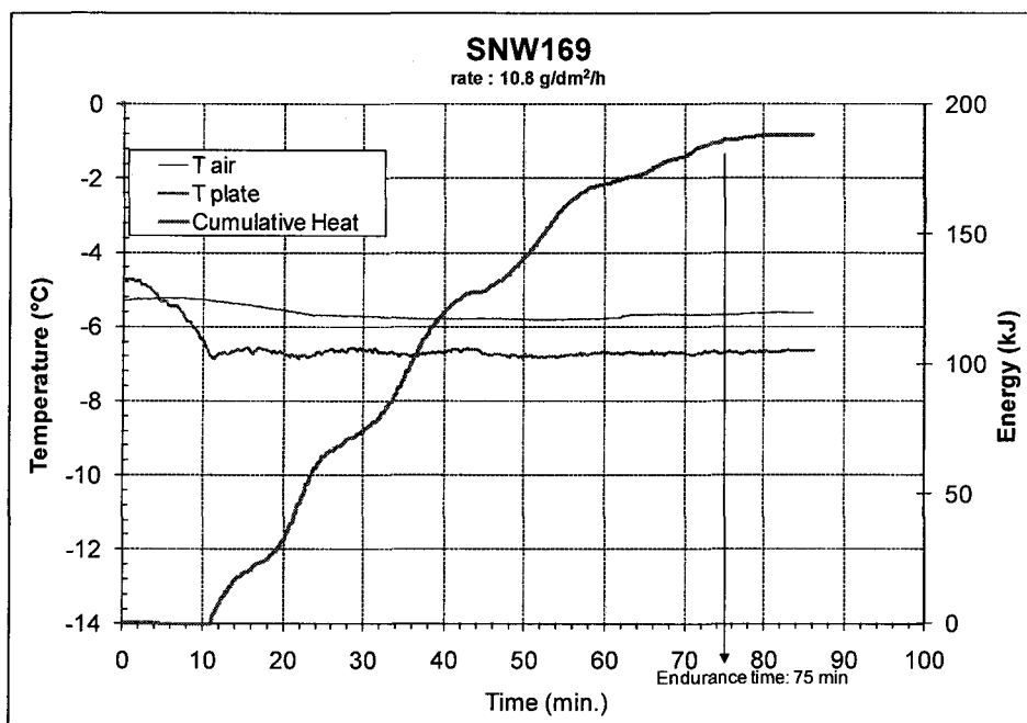
Figure 9 : Température de l'air et de la plaque enregistrée durant un essai (LIMA 2004), [22]
