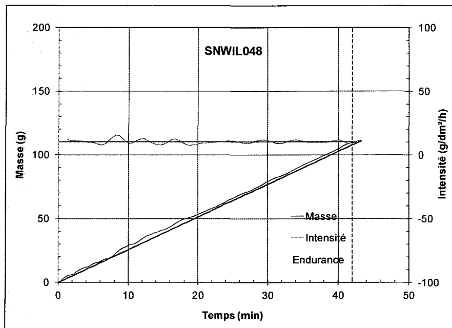
Figure A-10 : Évolution de la masse et de l'intensité des précipitations de neige au cours d'un essai de la condition 4 avec une boîte à neige à petits trous, essai SNWIL048
