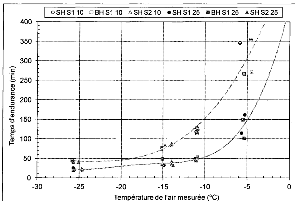
Figure 84 : Temps d'endurance pour les différents essais
