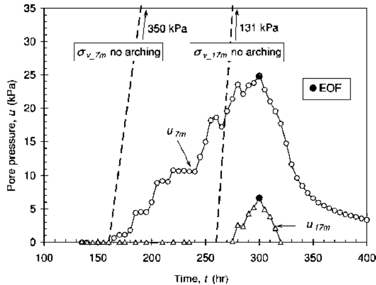
Figure 2–37: Résultats des mesures de pression à la mine Savannah Nickel (Helinski et al., 2010)
