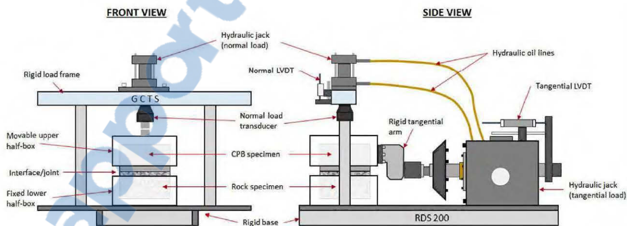
Figure 3–6 Appareil de cisaillement GCTS RDS 200 (Koupouli et al., 2016)
