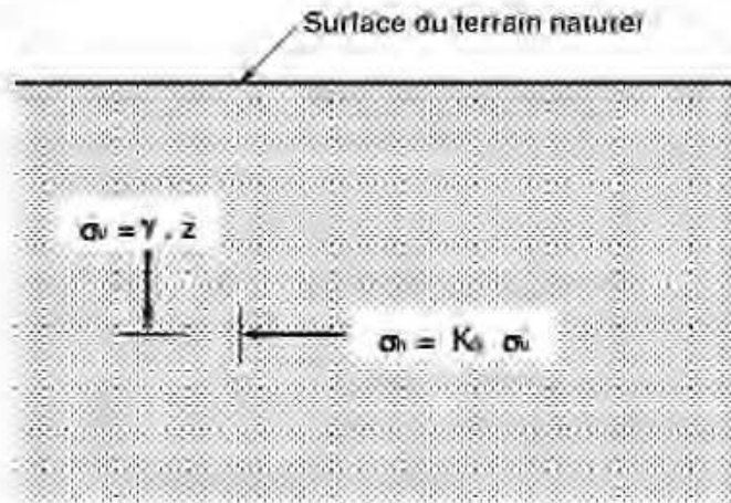
Figure 2-30 Représentation schématique du coefficient de pression latérale des terres au repos
