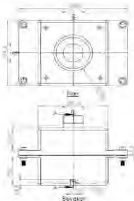
Figure 3-5 Coupe longitudinale et transversale du moule (d'après Plastique G+)
