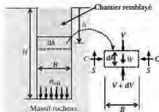
Figure 2-32 Chantier vertical étroit avec les forces agissant sur une couche horizontale (Aubertin et al., 2003)
