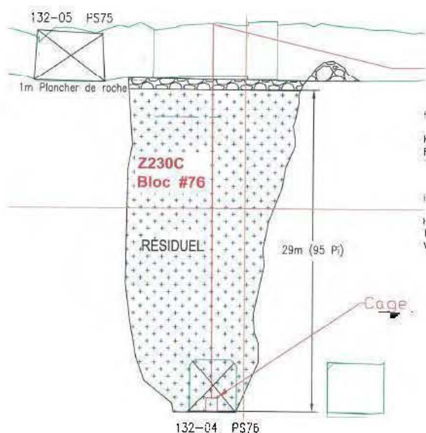
Figure 3-30 Coupe longitudinale du chantier #76 remblayé après son instrumentation
