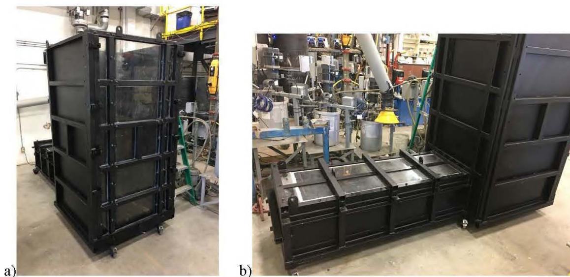
Figure 3-8 Images du modèle physique de chantiers miniers montrant a) une vue avant au niveau du chantier et b) une vue en arrière au niveau de la galerie
