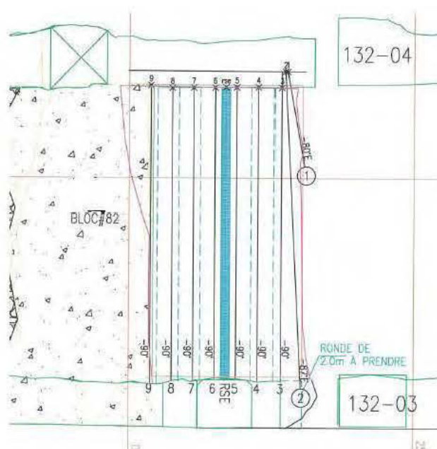
Figure 3-20 Coupe longitudinale du bloc 83, 132-03 au 132-04 Z230C (mine Westwood)
