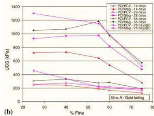
Figure 2-10 Effet du pourcentage des particules très fines sur la résistance du RPC (Fall et Benzaazoua 2005)
