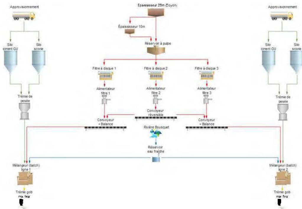
Figure 2–22 Schéma de fonctionnement ( flowsheet ) de l'usine à remblai de la mine Westwood
