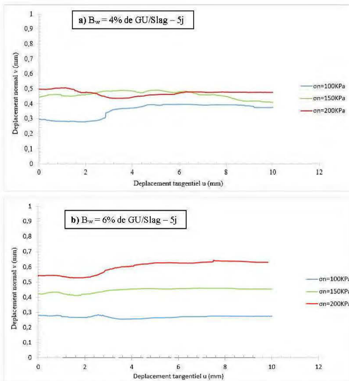
Figure 4-4 Courbes de déplacement normale-déplacement tangential des blocs de remblai curés à 5 jours avec a) 4% de liant, et b) 6% de liant
