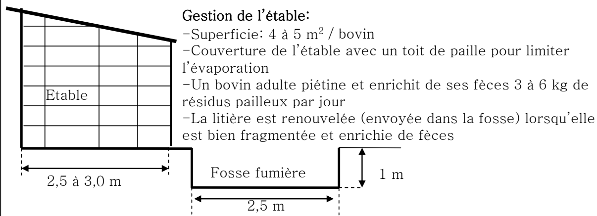
Figure 15 : Modèle d'étable fumièr avec fosse juxtaposée en zone de pluviosité supérieure à 600 mm / an (Berger, 1996)
