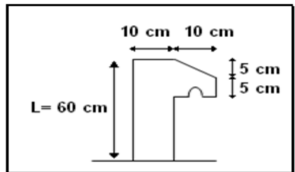
Figure IV.5 Schéma de l'acrotère Type1
