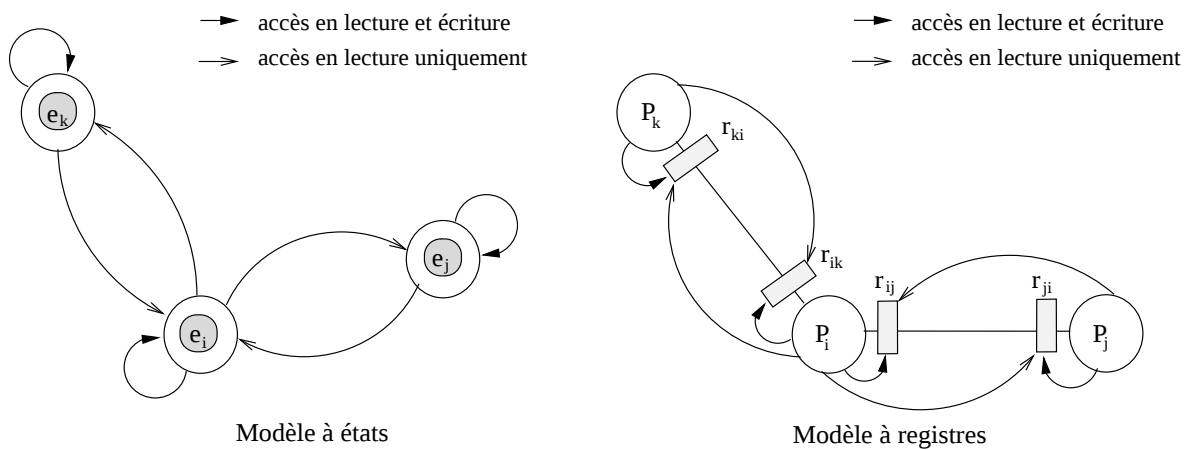
FIG. 1.1 – Modèles de communication par mémoires partagées.
