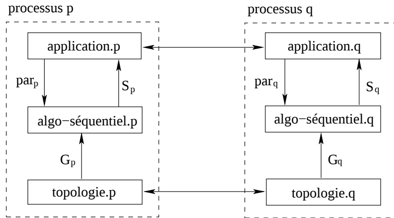
FIG. 4.4 – Transformateur général.
