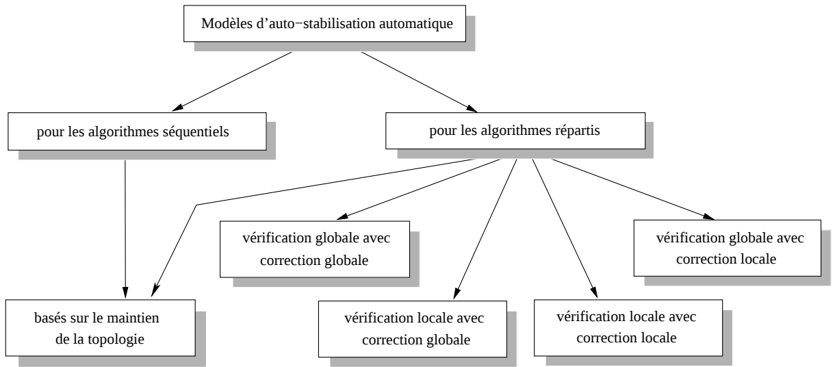
FIG. 3.1 – Classification des modèles d'auto-stabilisation automatique.
