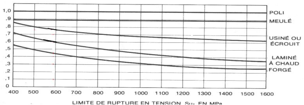
Figure III.12 : Facteur de fini de surface de source
