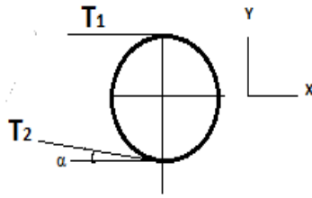
Figure III.2 : Tensions T_1 et T_2 du tambour d'entraînement
