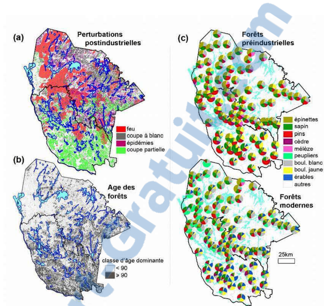
Figure 5.1 Cartes des principales perturbations post-industrielles (a) et de l'âge actuel des forêts (b) reconstituées à partir des cartes écoforestières du 4 e décennal. Les cartes (c) montrent les changements la fréquence d'occurrence de chaque taxon par district écologique pour les époques préindustrielle et actuelle (voir méthodes chapitre IV). Notez que dans la carte (a), la cartographie écoforestière ne prend pas en compte les perturbations partielles anciennes (coupes et épidémies de la première moitié du XX e siècle.).
