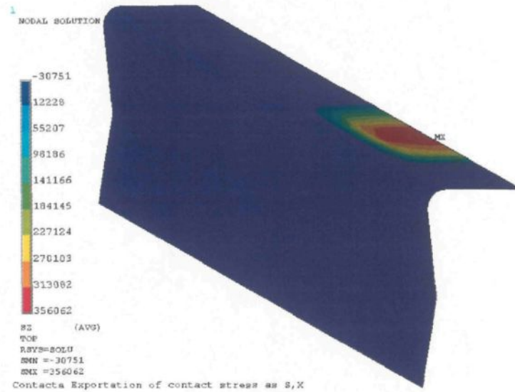
Figure 5.27 – Contrainte normale de contact sur l'interface entre le carbone et la fonte t = 4 heures (en Pa, méthode de pénalisation)
