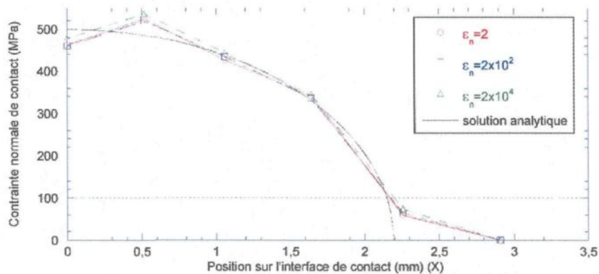
Figure 5.7 – Contrainte normale de contact t_n avec la méthode du lagrangien augmenté adapté (maillage 4 et comportement élastique)
