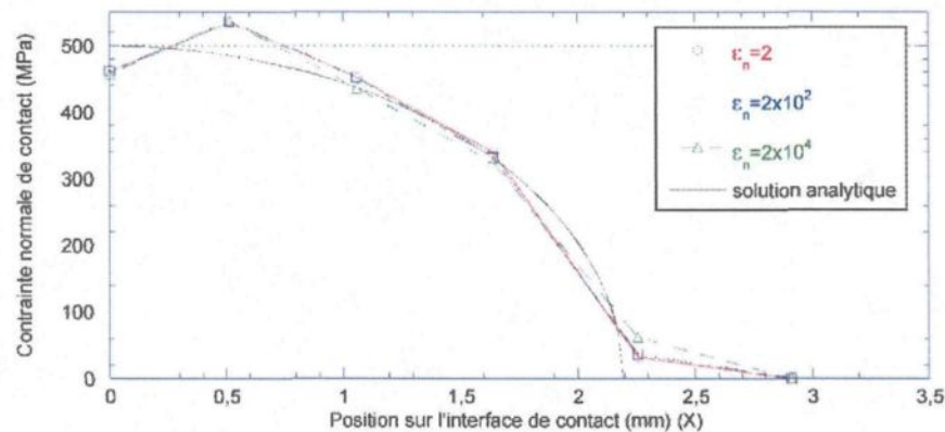
Figure 5.5 – Contrainte normale de contact t_n avec la méthode de pénalisation adaptative modifiée (maillage 4 et comportement élastique)
