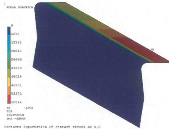
Figure 5.30 – Contrainte normale de contact sur l'interface entre le carbone et la fonte t = 6 heures (en Pa, méthode du lagrangien augmenté adapté)
