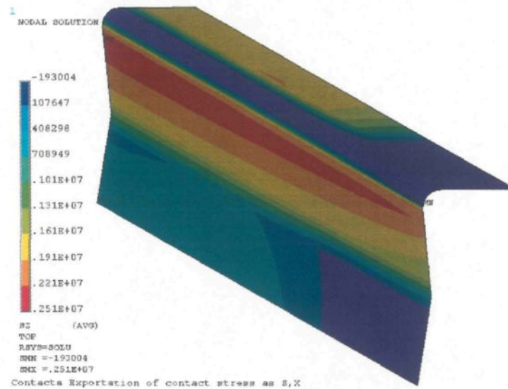
Figure 5.41 – Contrainte normale de contact sur l'interface entre le carbone et la fonte t = 18 heures (en Pa, méthode de pénalisation, hors équilibre)
