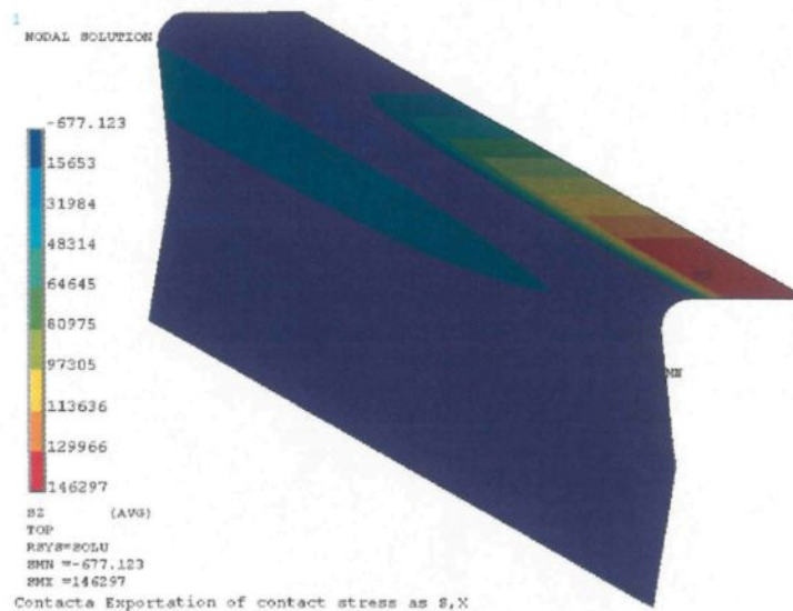
Figure 5.38 – Contrainte normale de contact sur l'interface entre le carbone et la fonte t = 14 heures (en Pa, méthode du lagrangien augmenté adapté)
