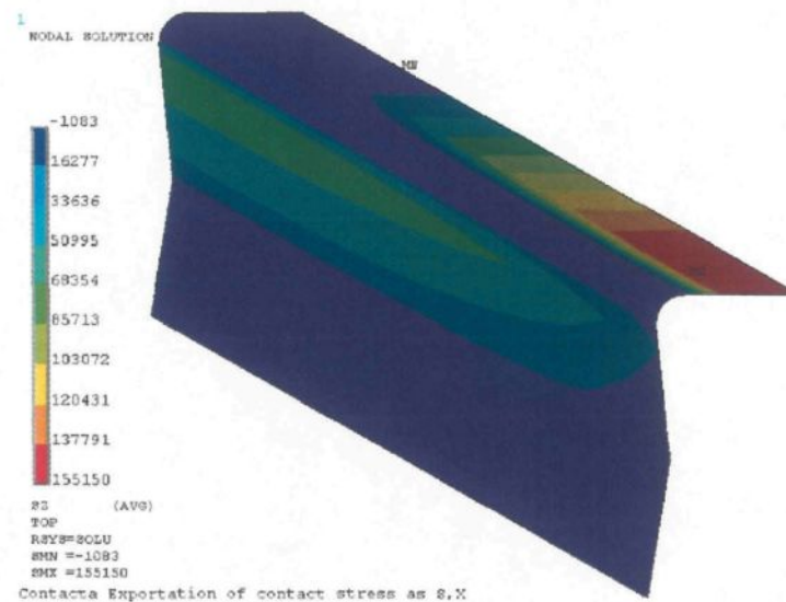
Figure 5.40 – Contrainte normale de contact sur l'interface entre le carbone et la fonte t = 16 heures (en Pa, méthode du lagrangien augmenté adapté)
