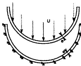
Figure 4.27 – Écrasement de deux tubes concentriques
