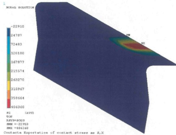
Figure 5.29 – Contrainte normale de contact sur l'interface entre le carbone et la fonte t = 6 heures (en Pa, méthode de pénalisation)
