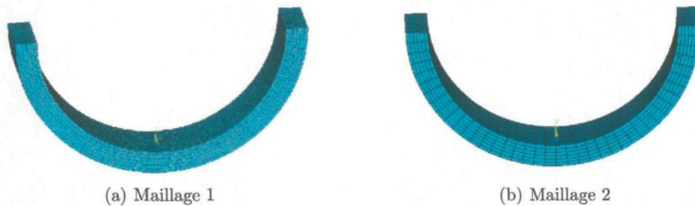
Figure 4.28 – Maillage des deux demi-tubes en trois dimensions.
