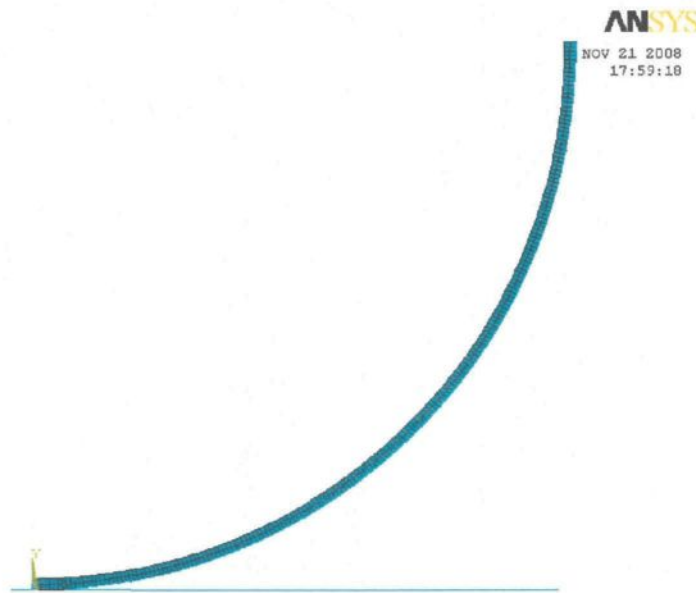
Figure 4.18 – Maillage du quart de tube en deux dimensions (maillage 200).
