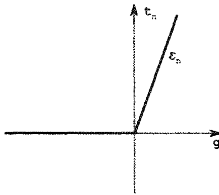
(a) Loi de contact unilatéral.
