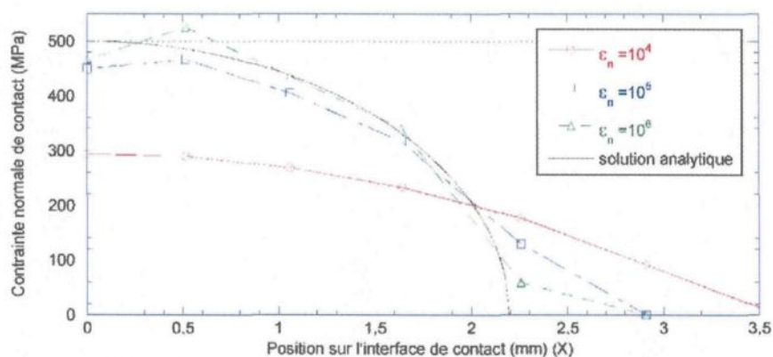
Figure 4.11 – Contrainte normale de contact t_n avec la méthode de pénalisation (mailage 4 et comportement élastique)
