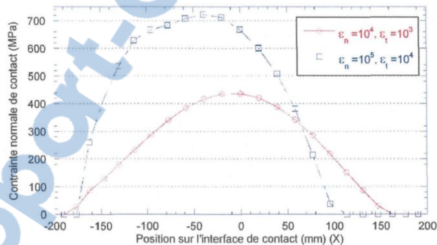
Figure 4.30 – Contraente normale de contact avec la méthode de pénalisation (maillage 2)
