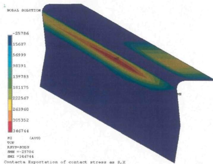
Figure 5.35 – Contrainte normale de contact sur l'interface entre le carbone et la fonte t = 12 heures (en Pa, méthode de pénalisation)
