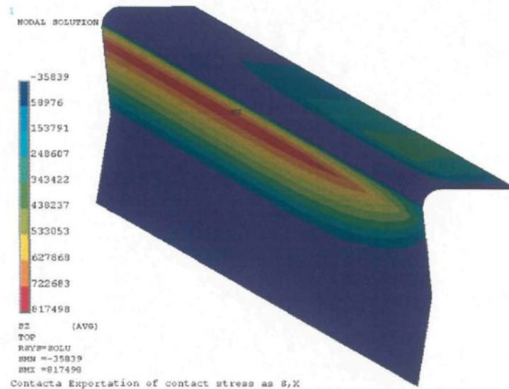
Figure 5.37 – Contrainte normale de contact sur l'interface entre le carbone et la fonte t = 14 heures (en Pa, méthode de pénalisation)
