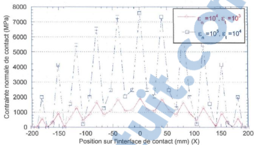
Figure 4.29 – Contraente normale de contact avec la méthode de pénalisation (maillage 1)
