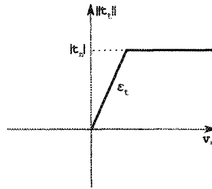
(b) Loi de frottement de Coulomb.
