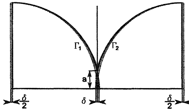
Figure 4.3 – Problème du contact de Hertz simplifié.
