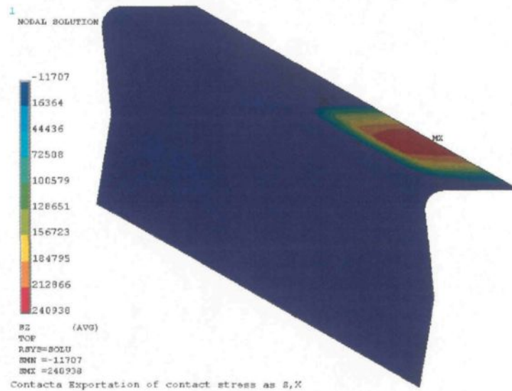
Figure 5.25 – Contrainte normale de contact sur l'interface entre le carbone et la fonte t = 2 heures (en Pa, méthode de pénalisation)
