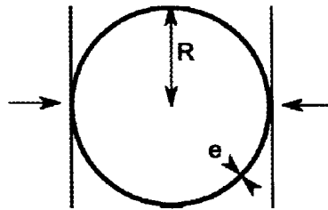
Figure 4.17 – Écrasement d'un tube entre deux plans rigides
