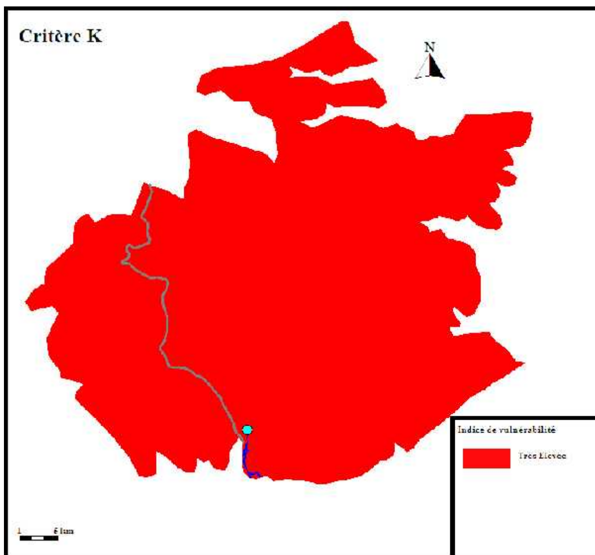
Figure V.6 : Indice de vulnérabilité selon le critère de Karstification.
