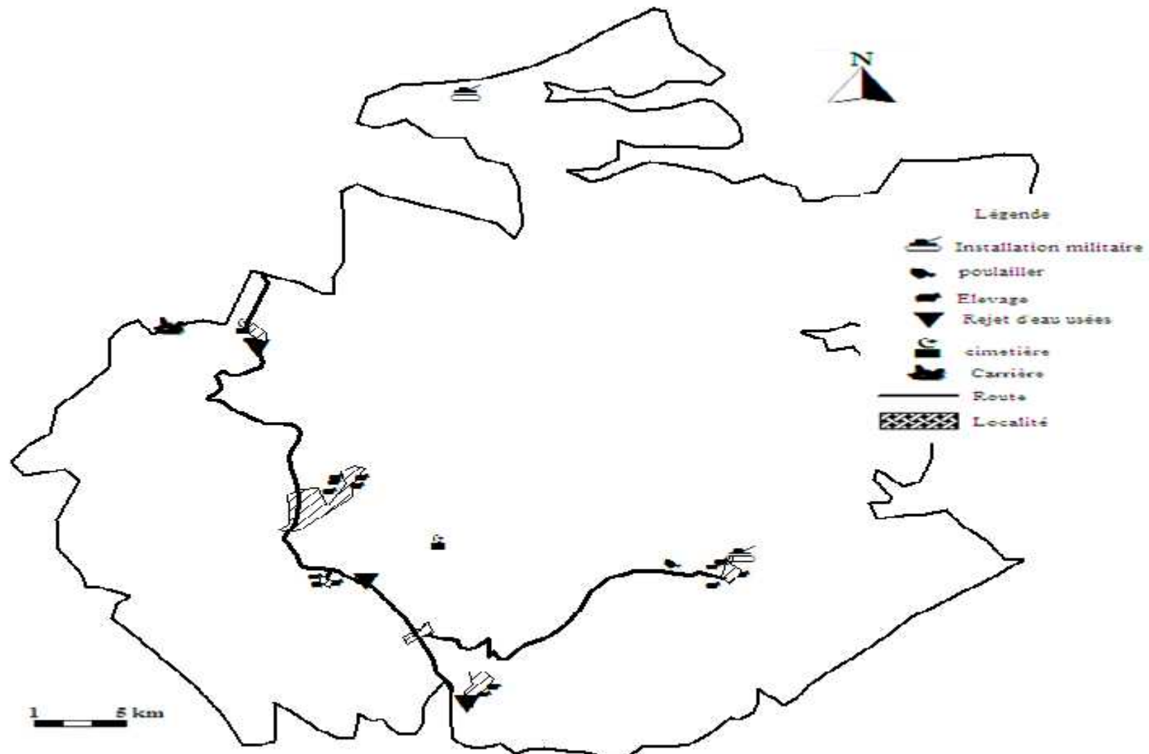
Figure V.9 : La carte d'aléas non classés
