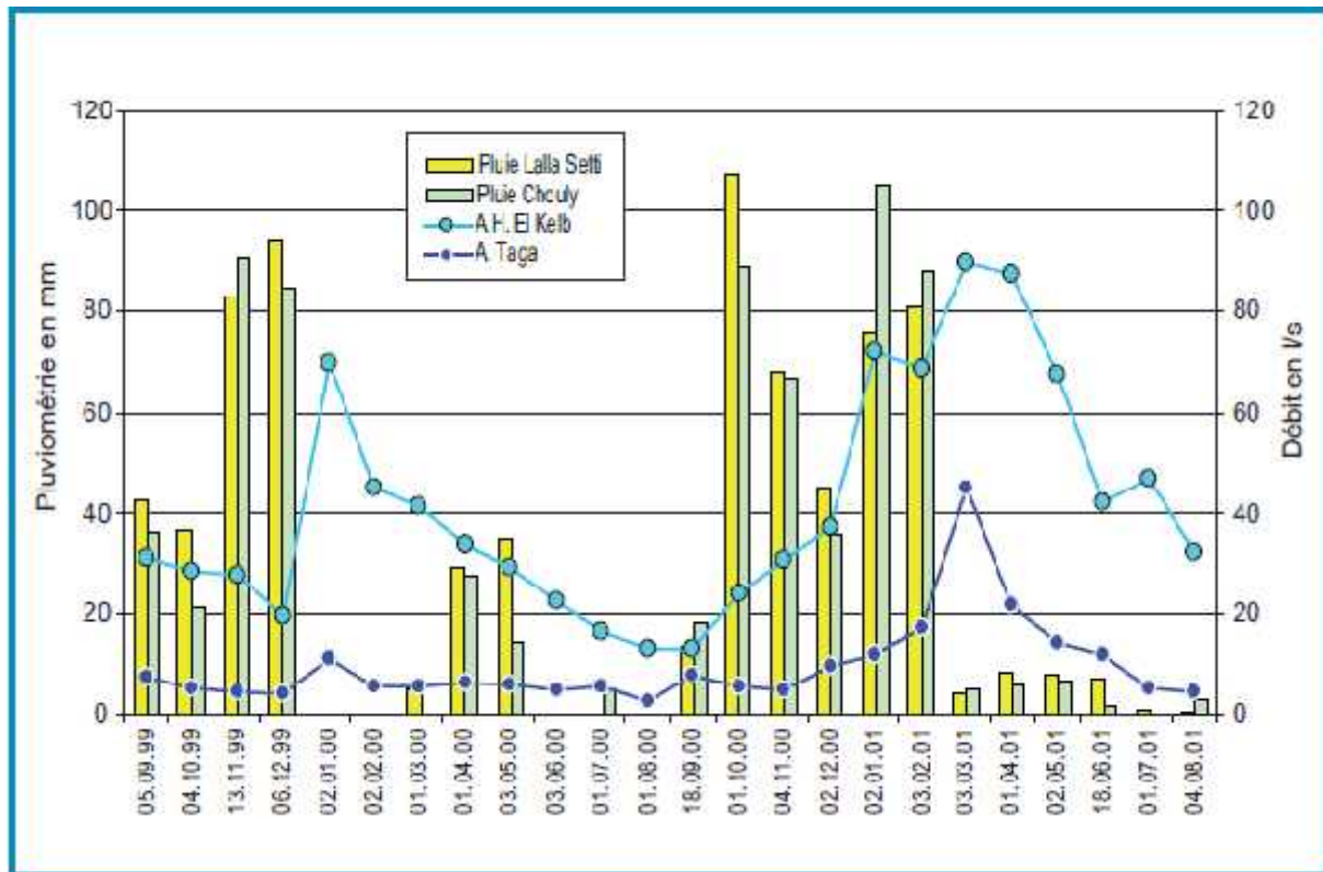
Figure IV.6 : Evolution du débit des sources de la Tafna avec la pluviométrie (1999-2001).
