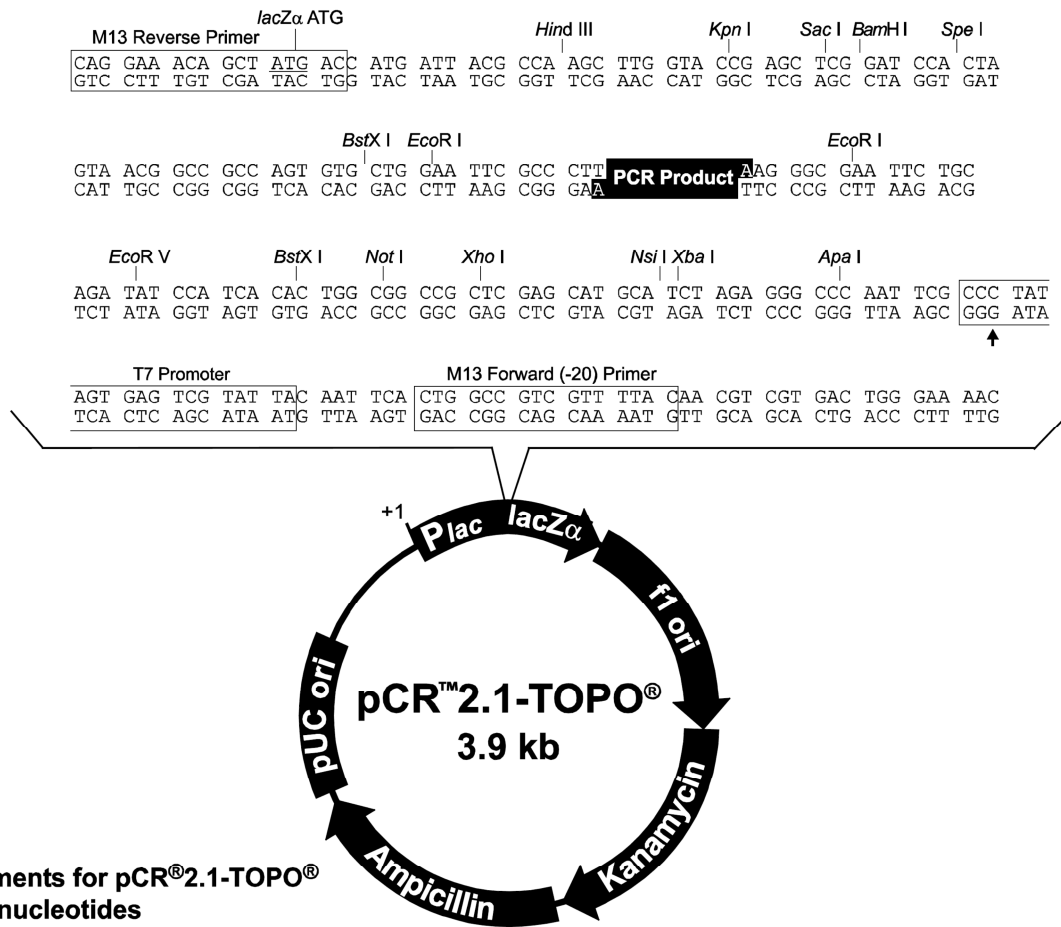
Figure 37 : Carte du vecteur pCR TM 2.1-TOPO ®
