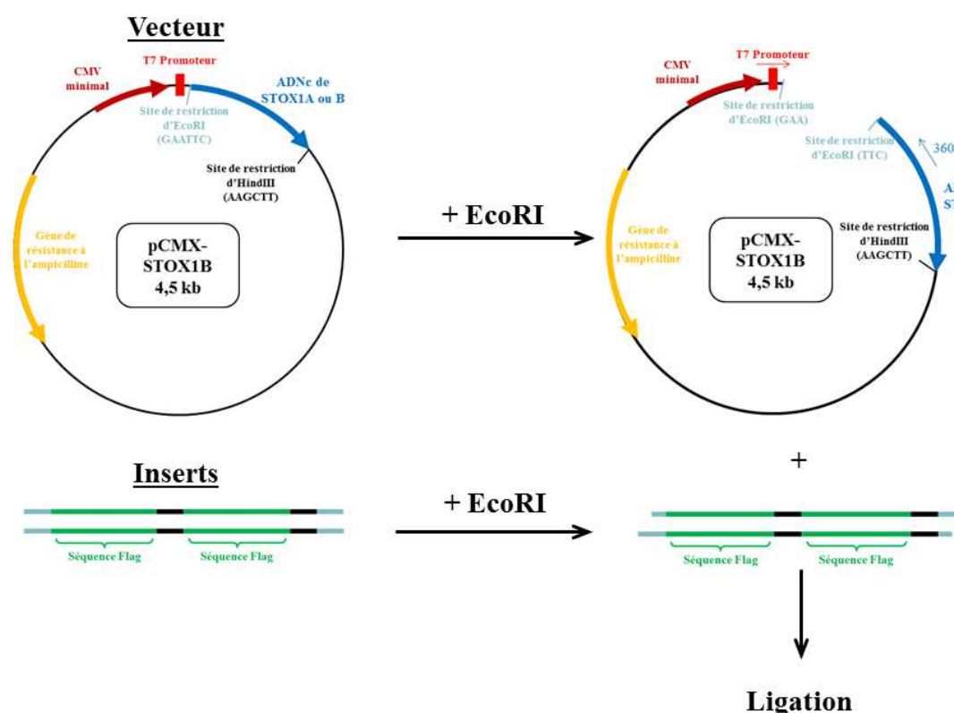
Figure 34 : Construction du vecteur Flag-STOX1
