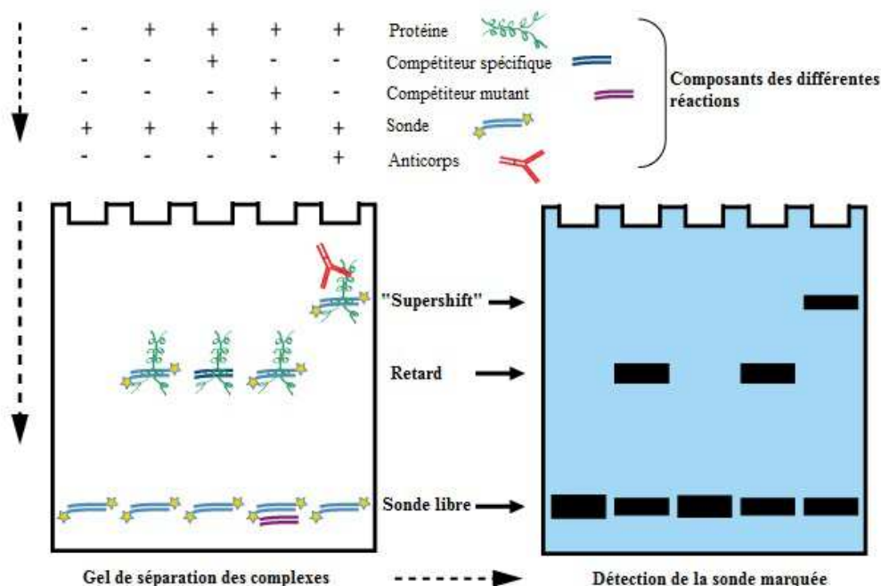
Figure 26 : Principe de l'expérience de retard sur gel
