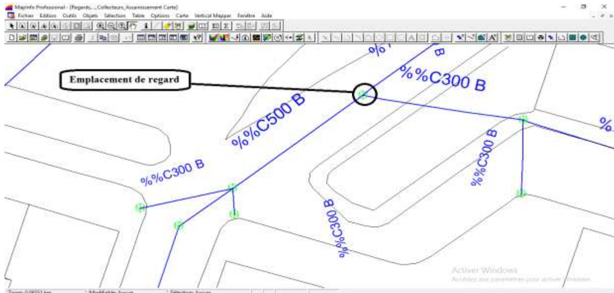
Figure IV.5 : Emplacement des regards sur les collecteurs
