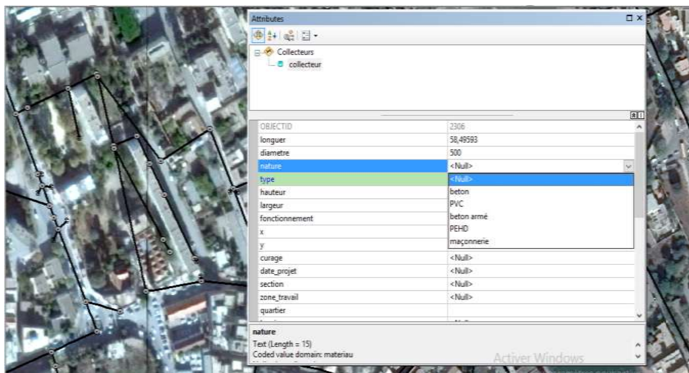
Figure B.4 : Domaine de la nature de matériau pour les collecteurs.
