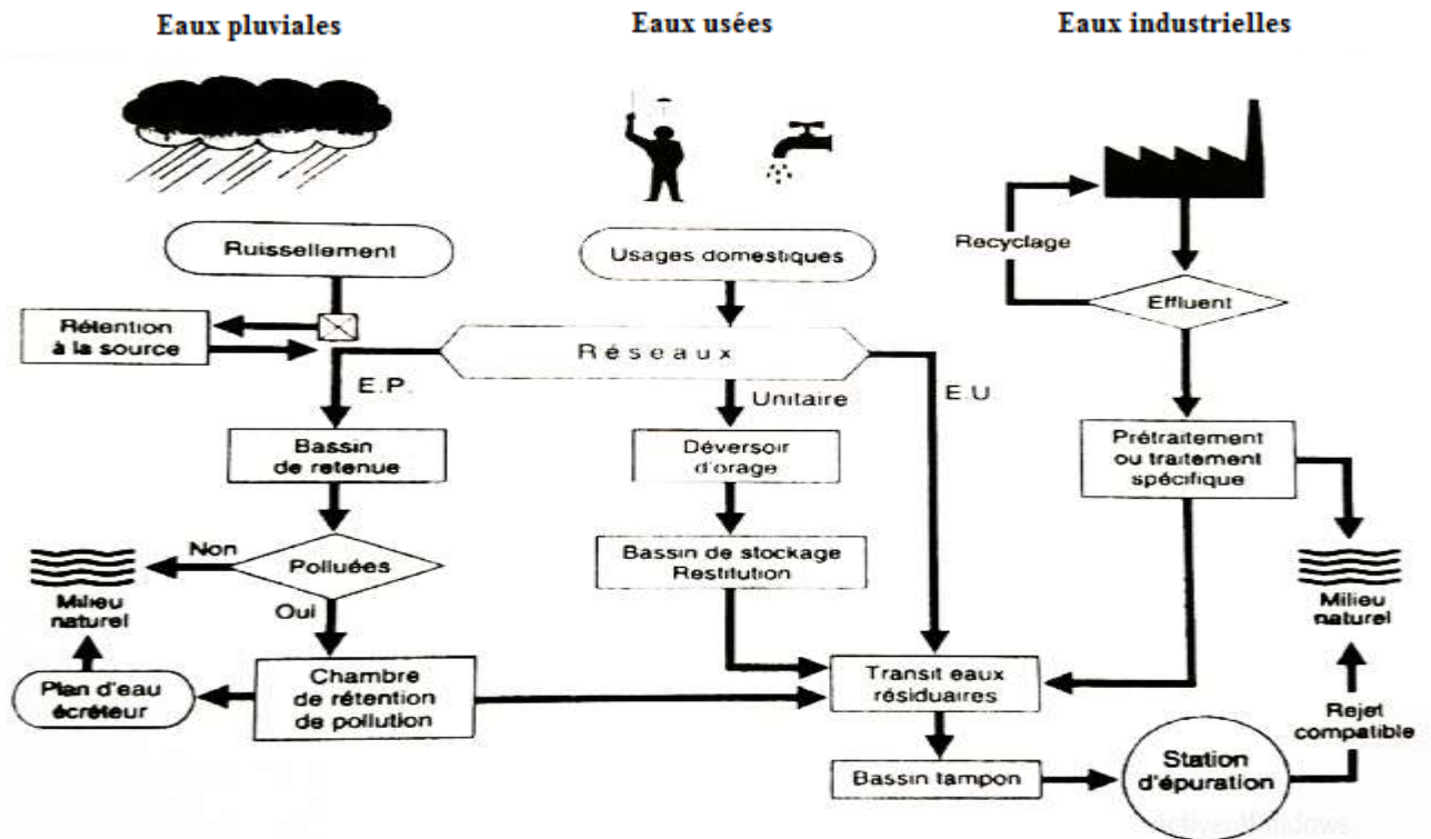
Figure I.1 : Structures fonctionnelles des réseaux et ouvrages[6]
