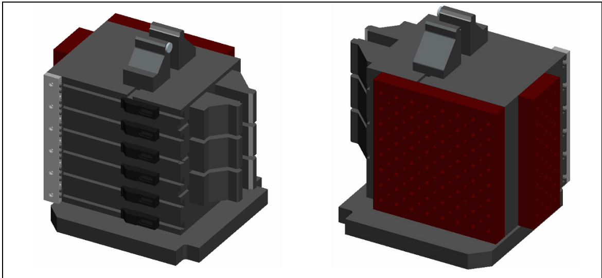
Figure 6.8 Représentation du montage d'usinage de la Makino A66.
