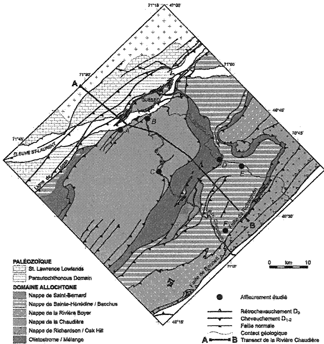
Figure 3 : Carte géologique de la zone de Humber externe dans la région du transect de la rivière Chaudière (Modifié de Sasseeville et al., 2008).
