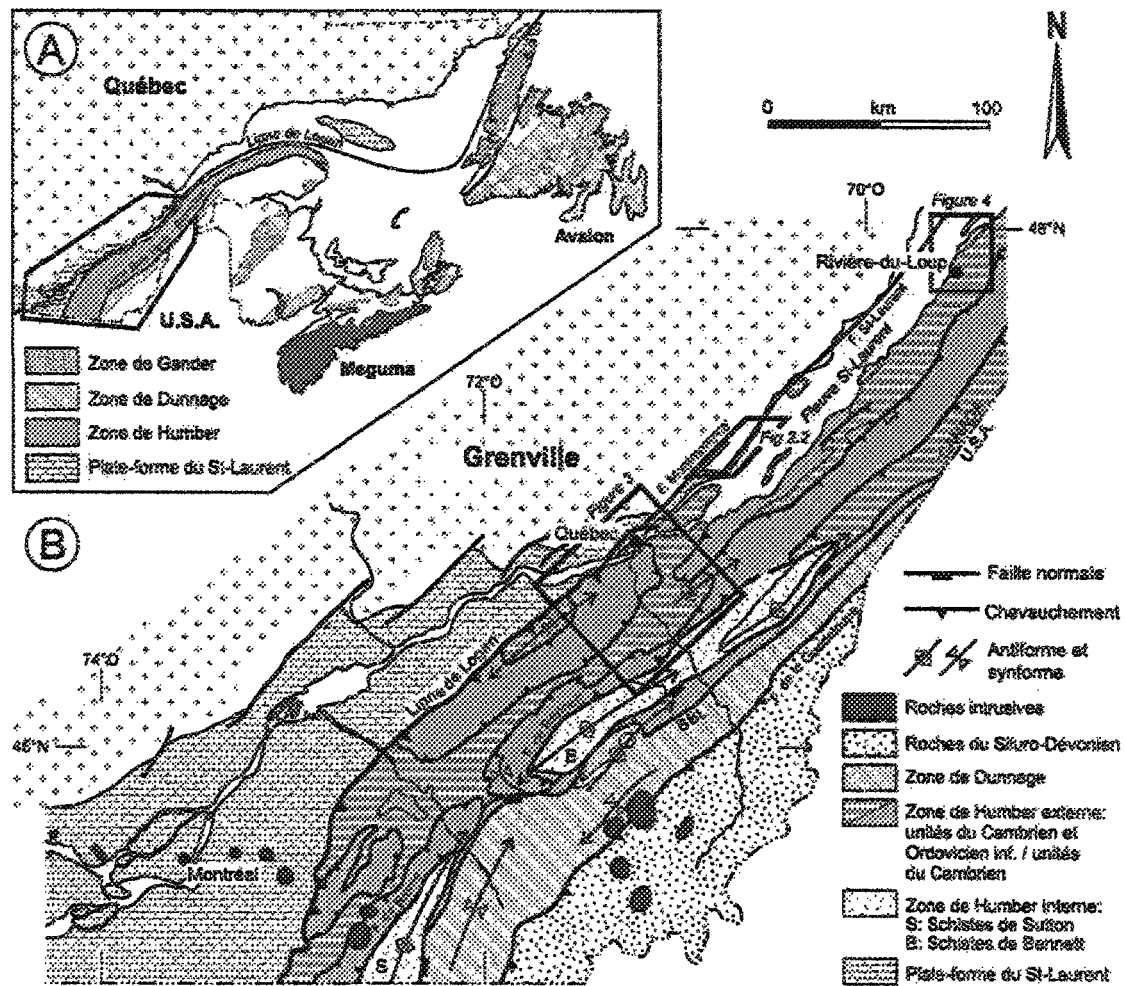
Figure 2 : Carte lithotectonique de la marge laurentine au Québec illustrant les secteurs étudiés dans le cadre de cette étude (Modifié de Sasseville et al., 2008).
