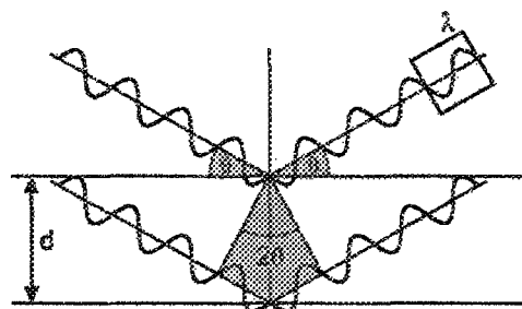
Figure 5: Loi de Bragg et la diffraction des ondes par les structures cristallines.
