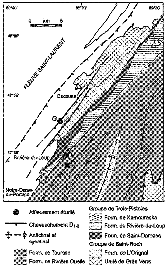
Figure 4 : Carte géologique de la nappe des Seigneuries dans la région du transect de Rivière du Loup (Modifié de Sasseville et al., 2008).
