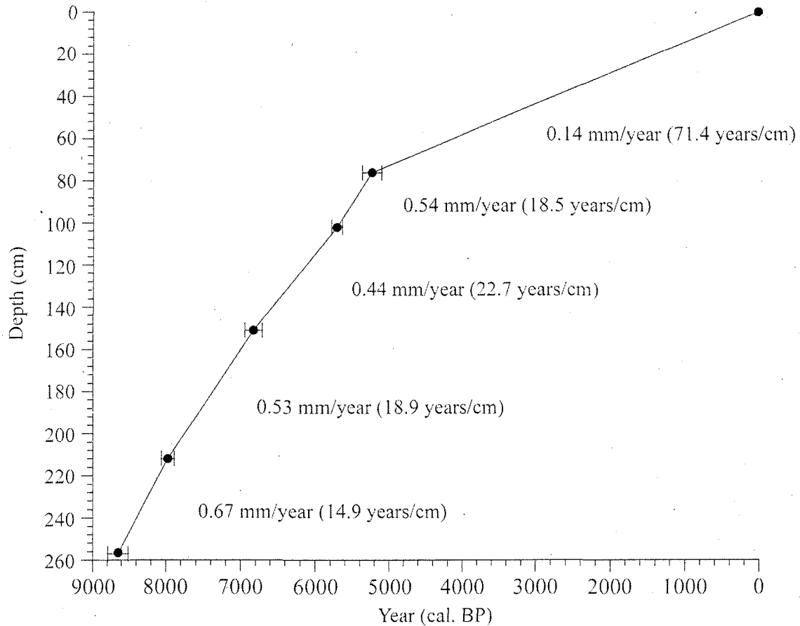
Figure 3.3 Peat accumulation rate for the Lac des Îlets peatland (Saguenay, Québec, Canada).
