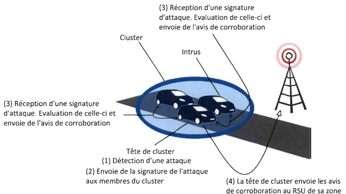
Figure 7: Processus de détection basé véhicule
