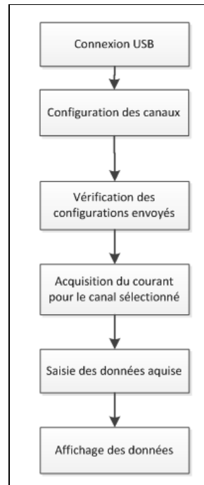
Figure 2.22 Étapes de la mesure de courant
