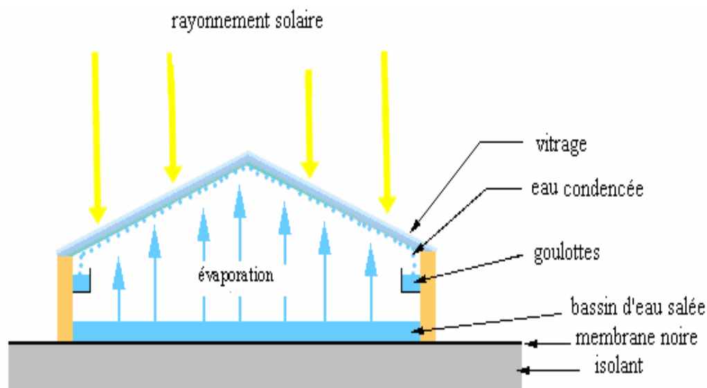
Figure II. 5 : Distillateur solaire à effet de serre [42].
