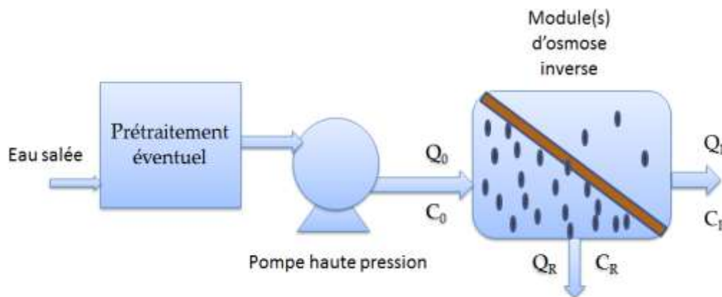
Figure II. 8 : Schéma de principe d'une unité d'osmose inverse [4].
