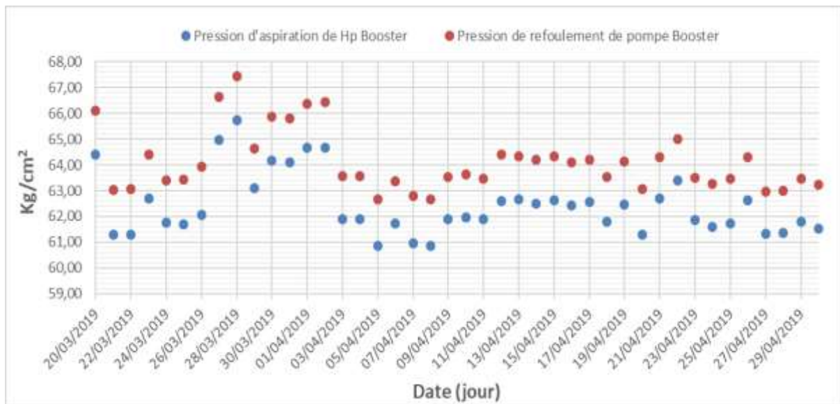
Figure V. 10 : Variation journalière des pressions de la pompe booster
