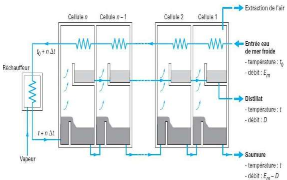
Figure II. 4 : Distillateur par détentes successives [3].
