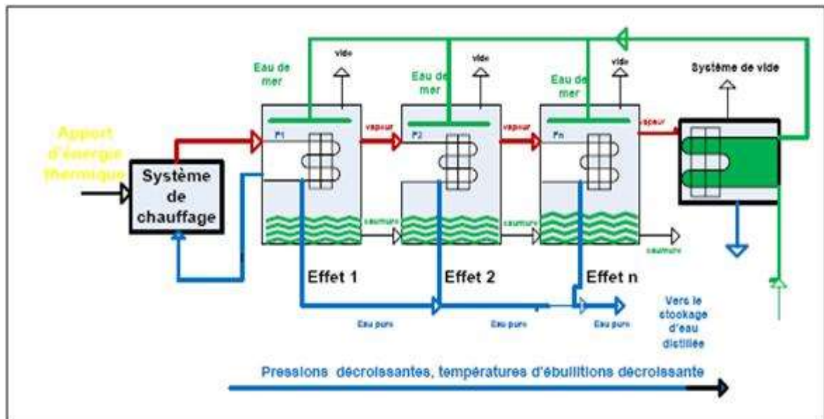
Figure II. 3 : Schéma de principe d'un système d'évaporateurs multiples effets (MED) [G].
