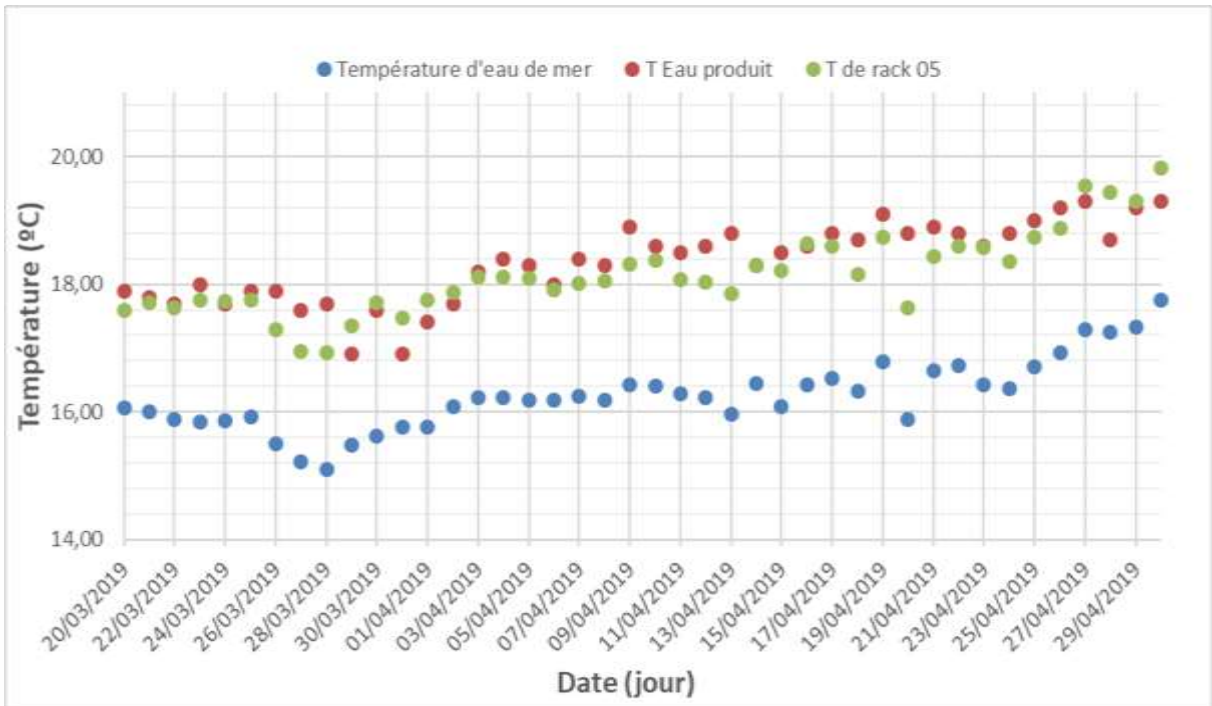
Figure V. 12 : Variation journalière de la température d'eau de mer, d'eau produite et d'eau dans le rack n°05 (Période entre le 20 Mars et le 30 Avril 2019).
