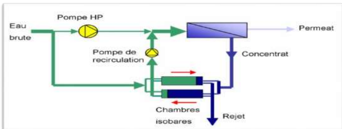
Figure III. 11 : Schéma de la récupération d'énergie [49].
