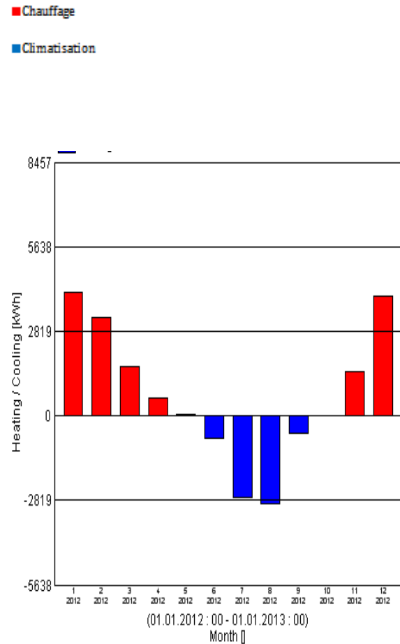
Figure 4-10 : la consommation énergétique du chauffage et climatisation d'un bâtiment isolée.
