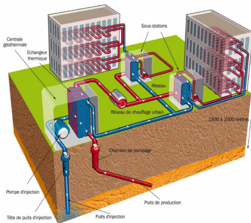
Figure 1-6 : Schéma d'une installation-type de géothermie (D'énergie renouvelables et leur exploitation ,2015).
