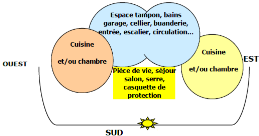
Figure 2-5 : L'implantation et l'orientation du bâtiment ou de la maison et des différentes pièces. (HESPUL, Les grands principes de l'architecture bioclimatique, 2015)
