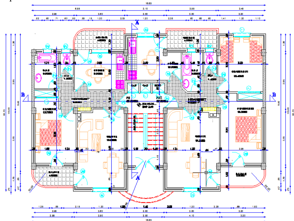
Figure 4-1 : Vue en plan du logement social à usage d'habitation.
