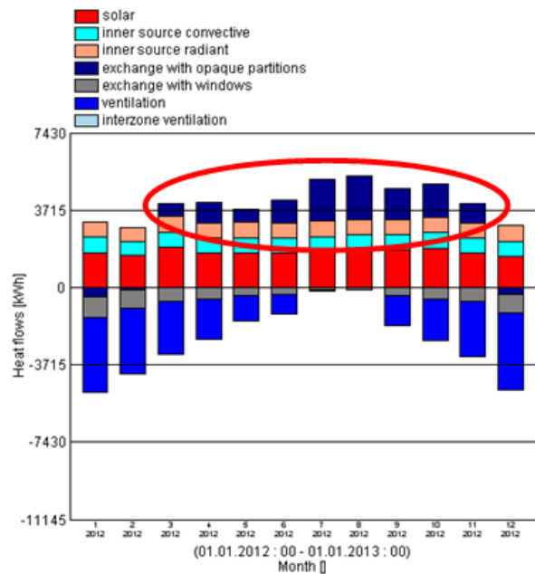
Figure 4-12 : les pertes et les gains énergétiques à travers les différents éléments de construction durant l'année d'un bâtiment isolée.
