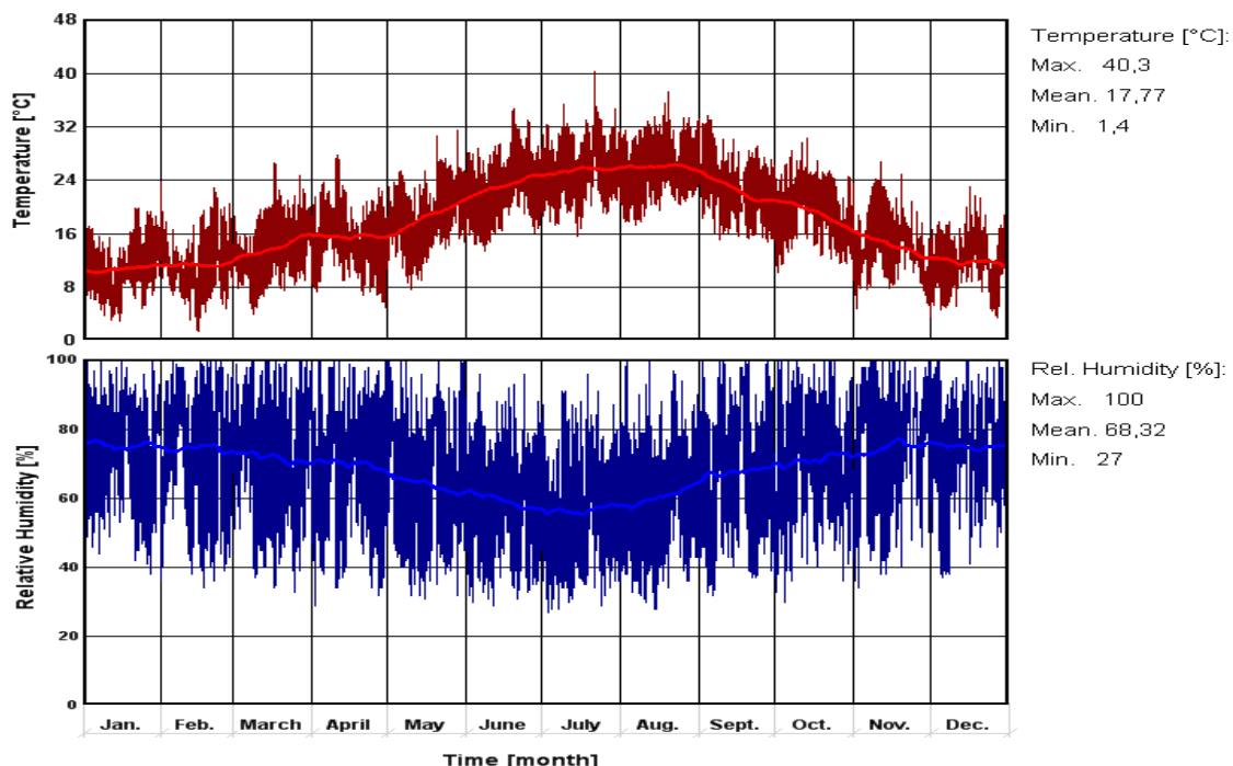
Figure 4-5: courbe d'humidité relative et de température extérieure du climat de Tlemcen analysées par Wufi.
