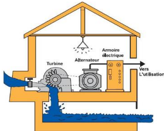
Figure 1-7: Centrale hydraulique, (Guide des Énergies Renouvelables, 2007).
