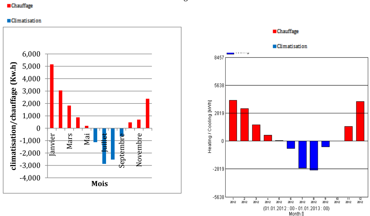
Figure 4-14 : Comparaison de la consommation énergétique (chauffage /climatisation) d'un bâtiment isolé.
