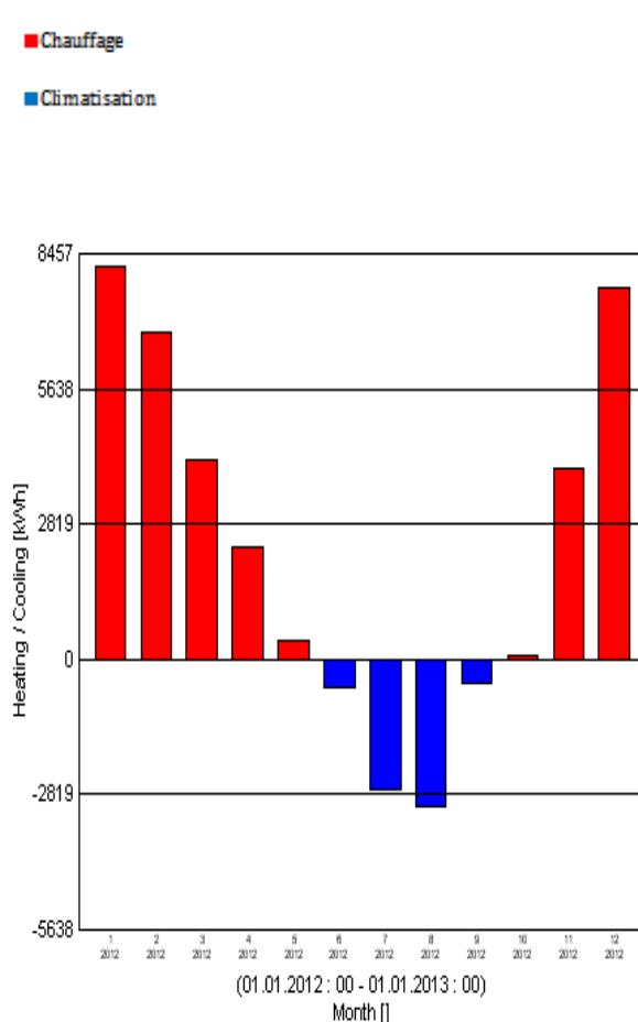
Figure 4-9 : la consommation énergétique du chauffage et climatisation d'un bâtiment énergivore.
