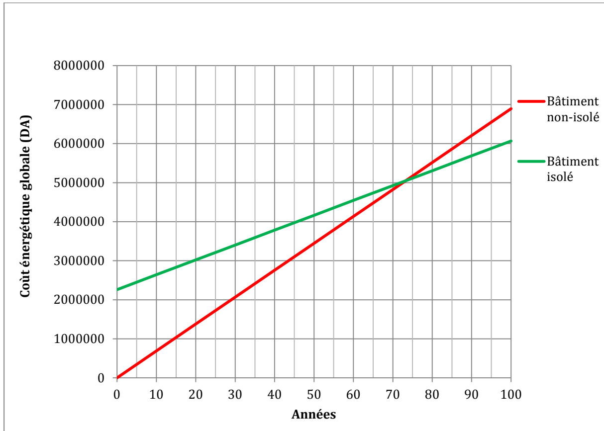
Figure 4-16 : Coût énergétique global sur une période de 100 ans avec un temps de retour sur investissement (TRI) de 73 ans (Chauffage au gaz et climatisation à l'électricité)
