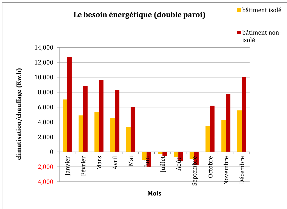
Figure 4-7 : comparaison entre les besoins des deux bâtiments pour T_{confort}
