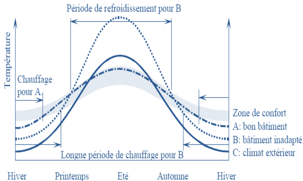
Figure 1-11 : Évolution des températures dans des bâtiments au cours de l'année, sans effet des installations techniques de chauffage ou climatisation (N.Morel et E.Gnansounou ,2008).
