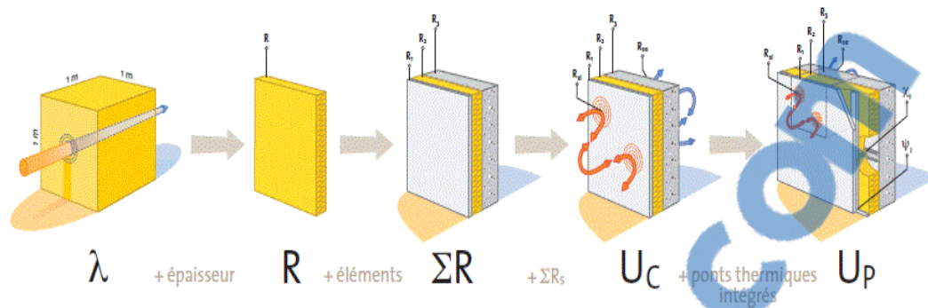
Figure 2-8 : Résumé des principales valeurs qui permettent de caractériser les performances thermiques d'une paroi opaque, (PLACO SAINT-GOBAIN ,2016)
