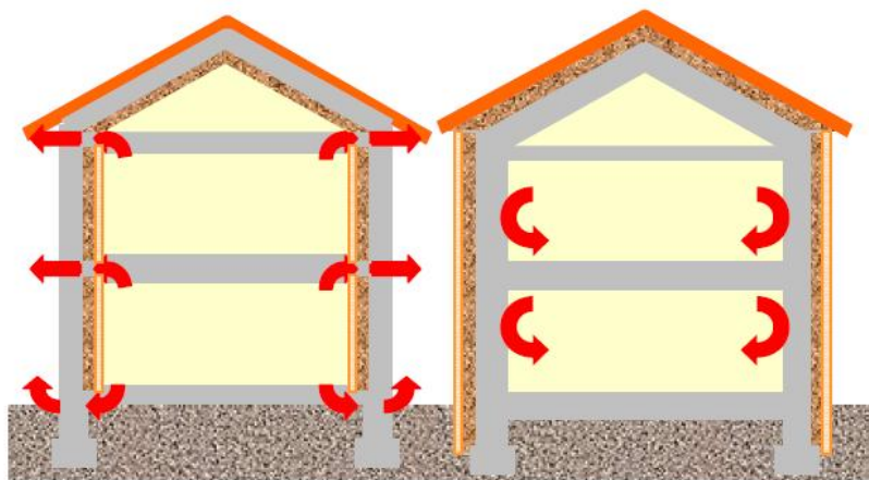
Figure 2-7 : A gauche, isolation intérieure : de nombreux ponts thermiques sont inévitables à chaque étage. A droite, isolation extérieure, entourant complètement la structure (N. Morel et E.Gnansounou . 2008)
