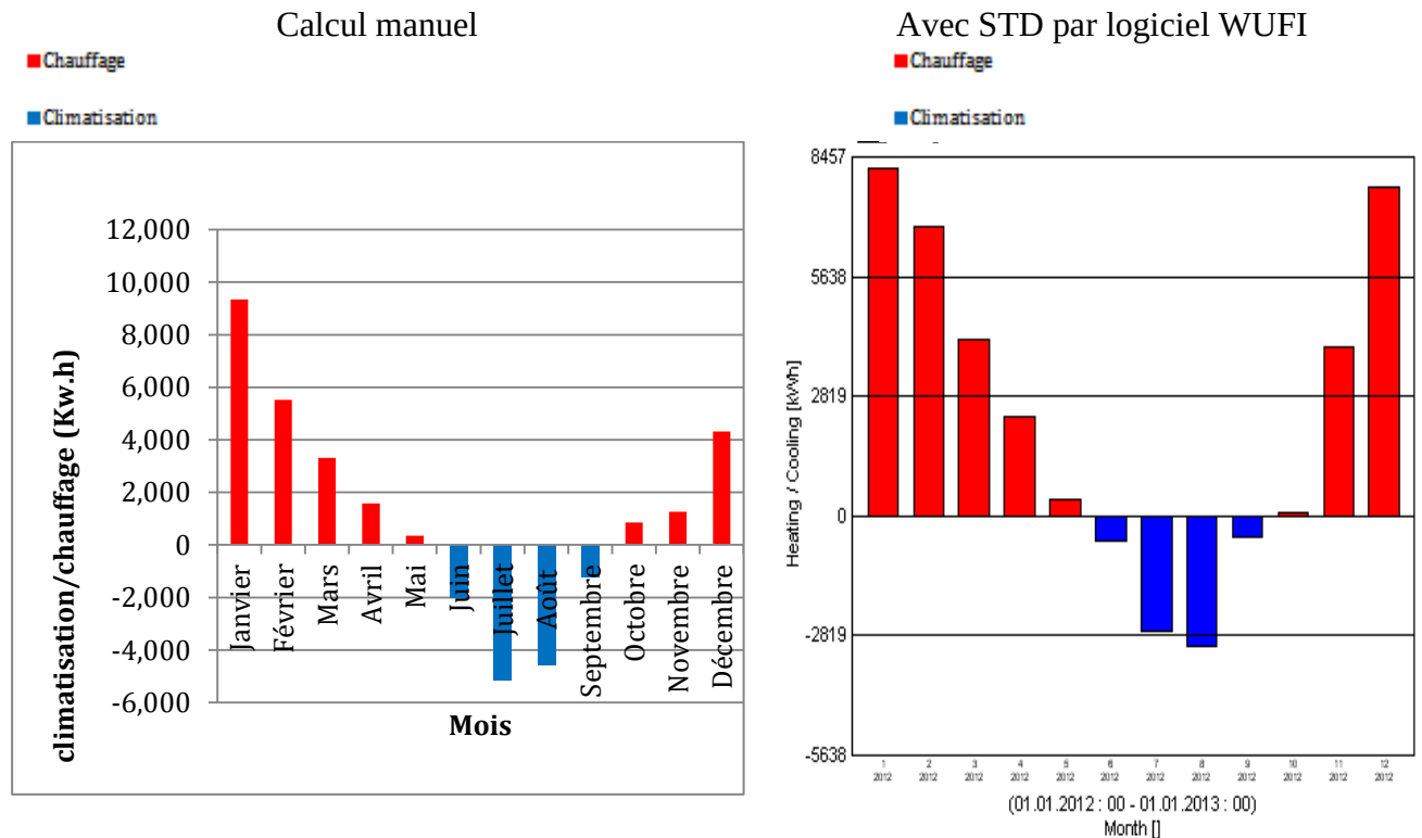
Figure 4-13 : Comparaison de la consommation énergétique (chauffage /climatisation) d'un bâtiment énergivore.
