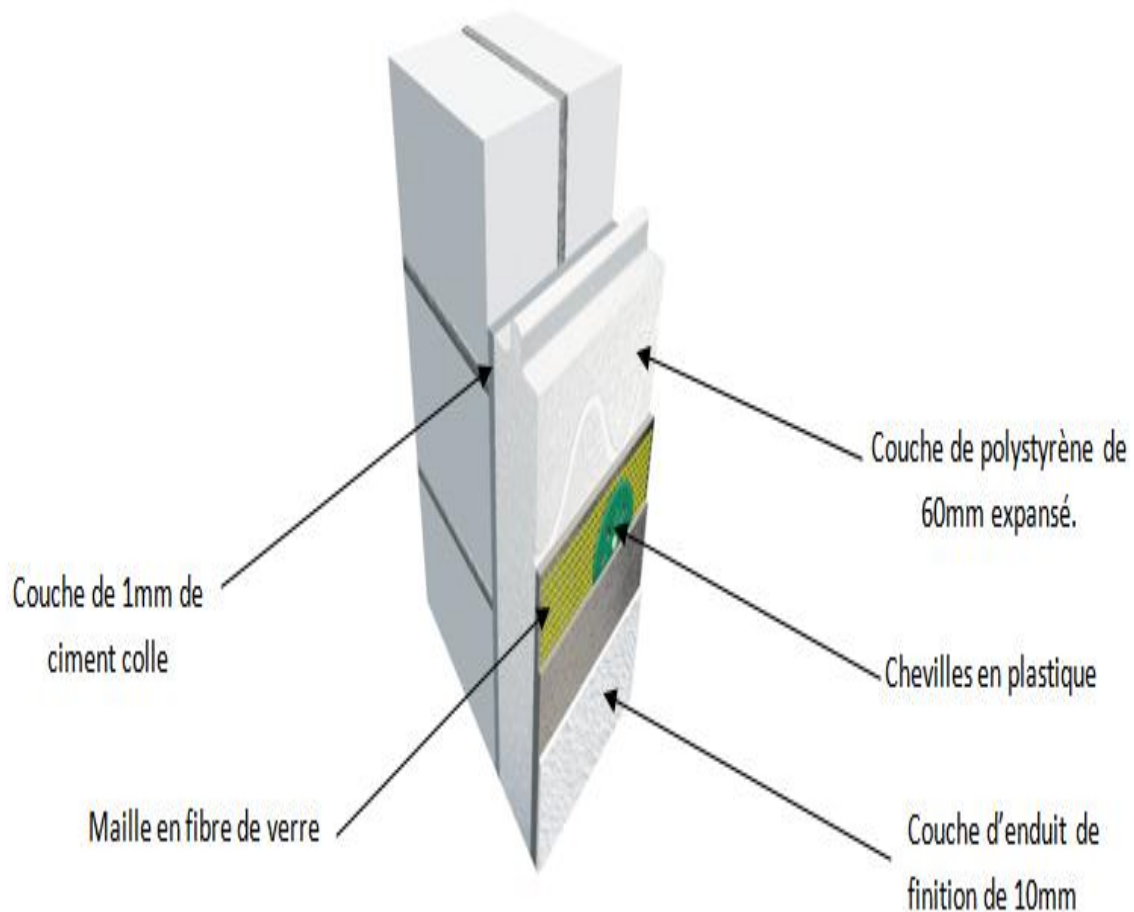
Figure 4-6 : Différents composants du Mur-chaud.
