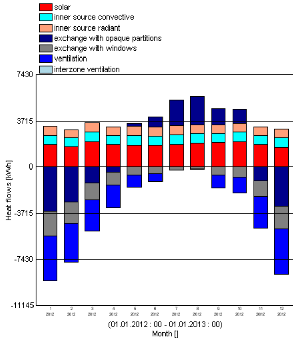
Figure 4-11 : les pertes et les gains énergétiques à travers les différents éléments de construction durant l'année d'un bâtiment énergivore
