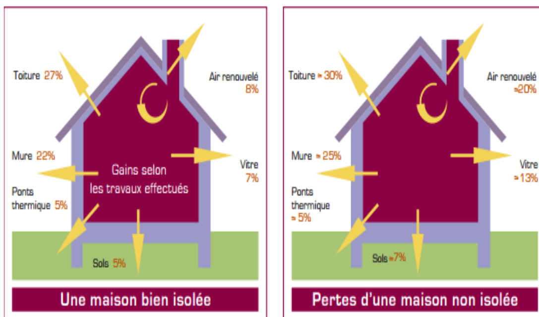
Figure 2-6 : Comparaison entre une construction bien isolée et non isolée (ADEME)
