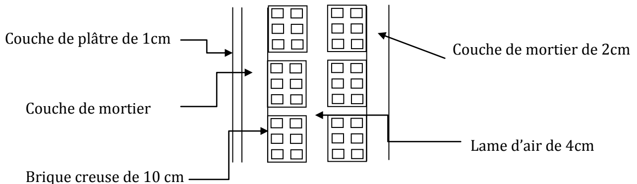
Figure 4-4 : Coupe transversal d'un mur double parois en brique creuse.
