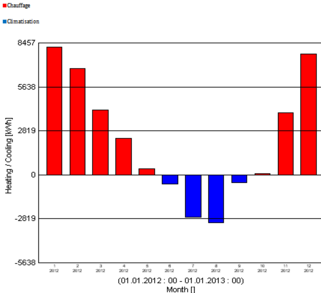
Figure 4-8 : la consommation énergétique du chauffage et du climatiseur en KWh durant l'année.
