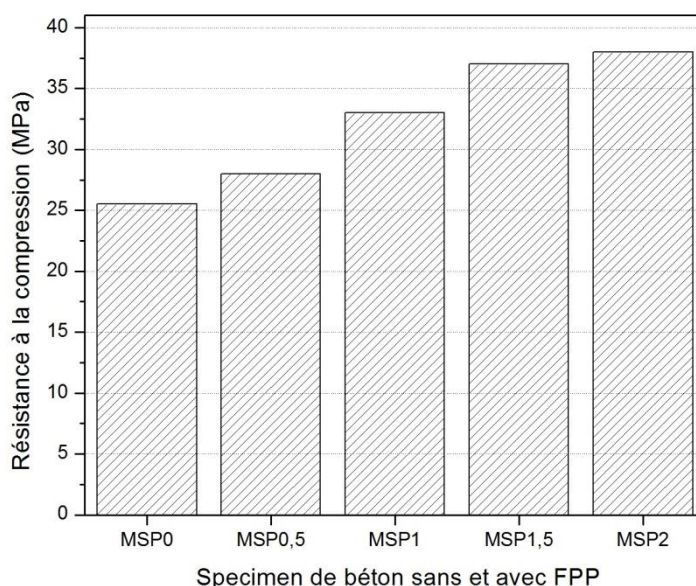
Figure II.6 : Résistance à la compression de différents échantillons de béton après 28 jours de durcissement (Kakooei et al., 2012)
