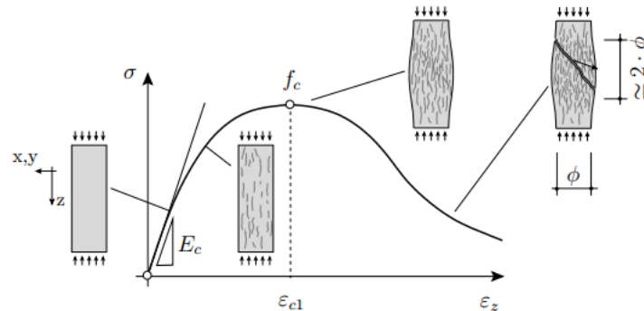
Figure I.10 : Représentation du comportement d'un cylindre en béton soumis à un effort de compression (Redaelli, 2009)
