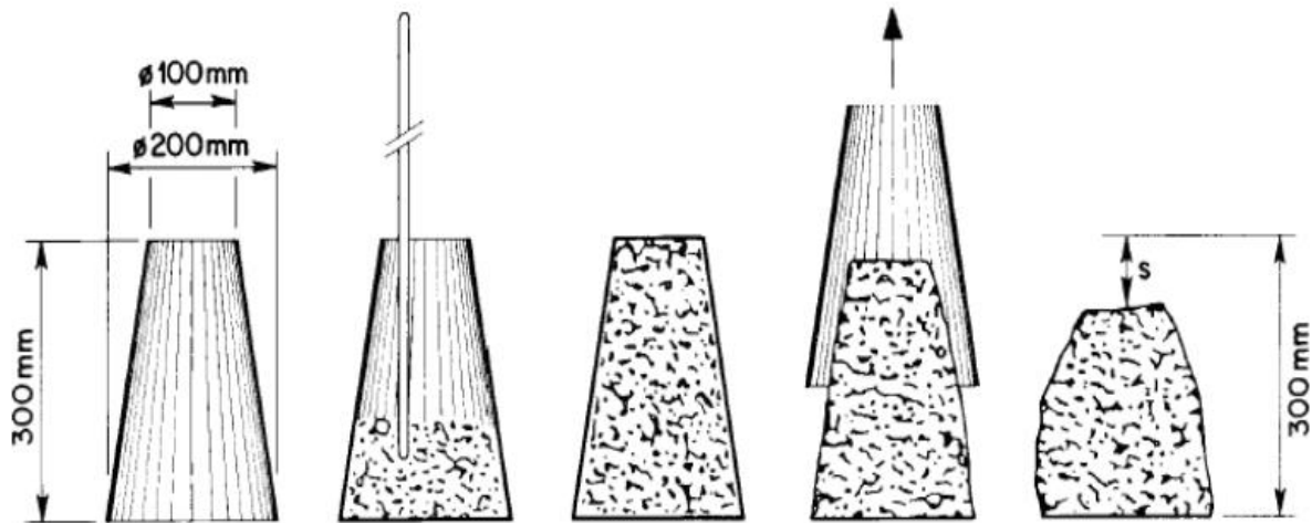
Figure III.5 : Les étapes de déroulement de l'essai d'affaissement au cône d'Abrams
