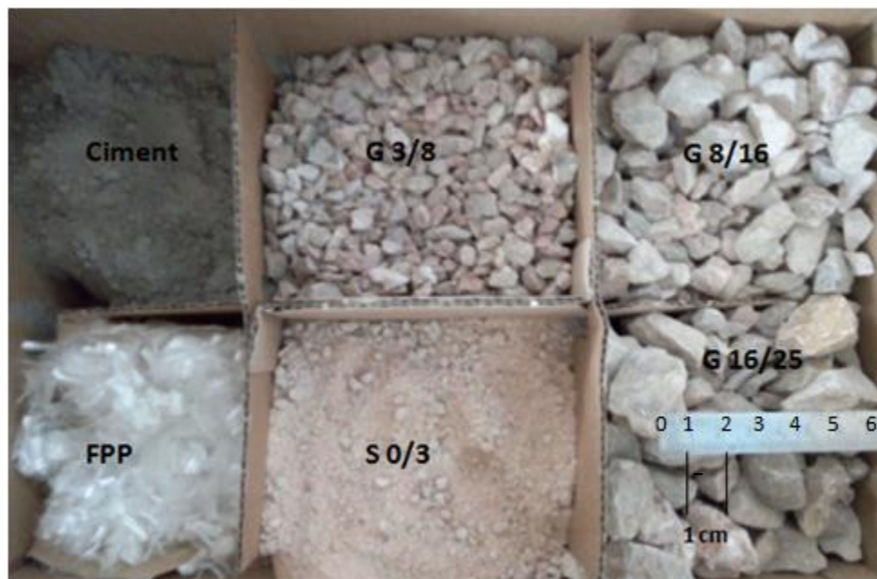
Figure III.1 : Photos sur les matériaux utilisés dans la préparation de nos bétons.
