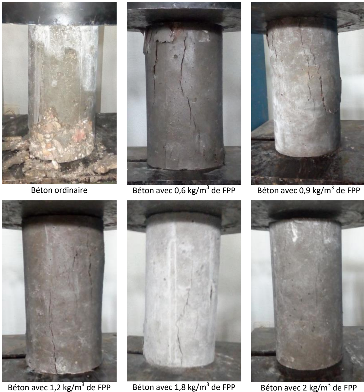
Figure IV.4 : L'influence des FPP sur le contrôle des fissures
