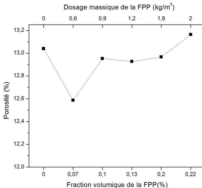
Figure IV.6: Pourcentage de la porosité de béton sans et avec la FPP.
