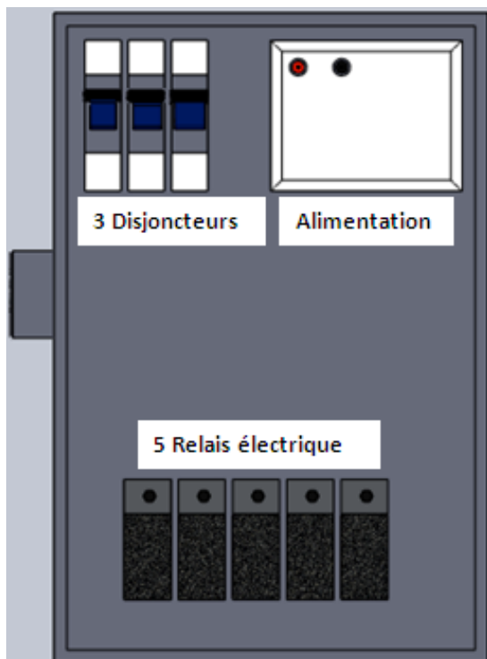
Figure 31: Vue interne du boîtier
