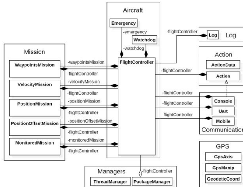
FIGURE 28: Architecture logicielle système embarqué
