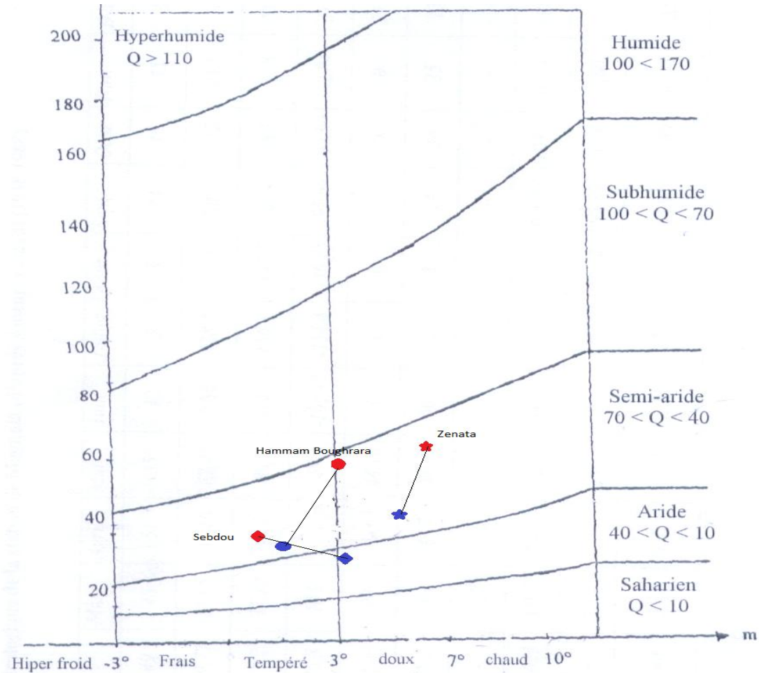
Fig 08 : Climagramme d'Emberger.
