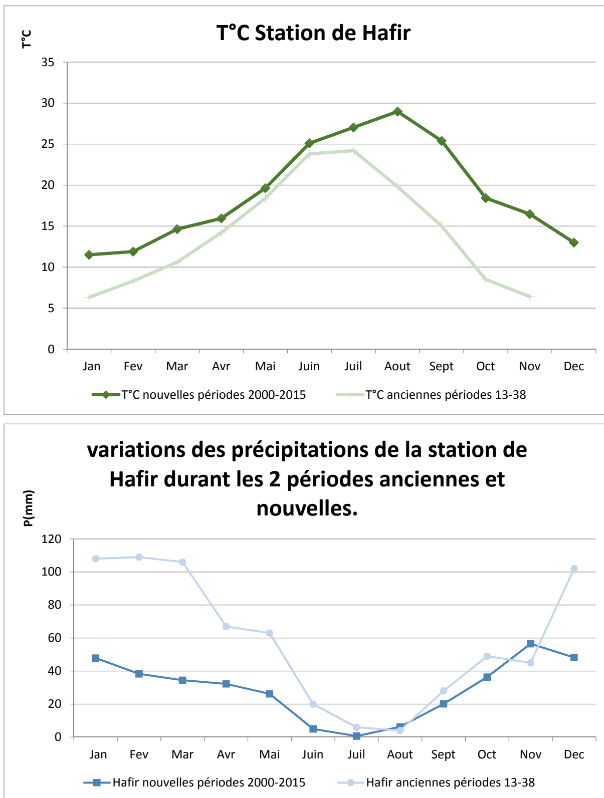
Figure2 : moyennes mensuelles des précipitations et des températures anciennes et nouvelles période (original).
