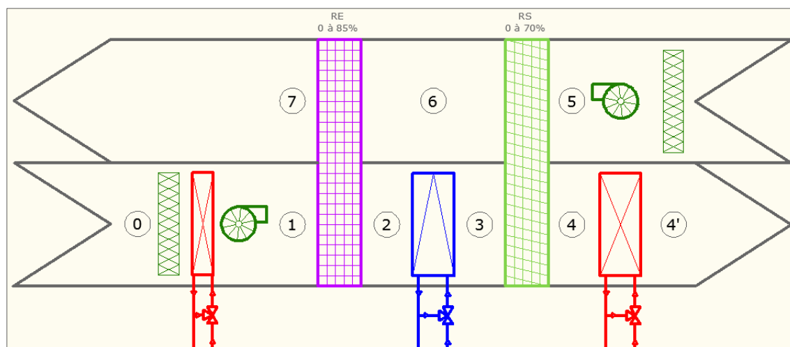
Figure 2.2 Système DOAS
