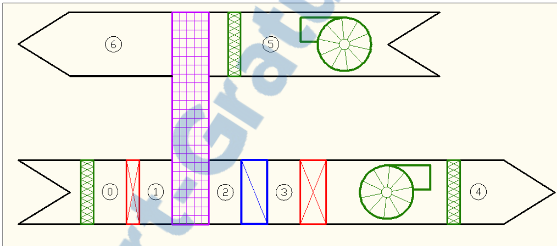
Figure 4.4 Système no4 : système à 100 % d'air frais
