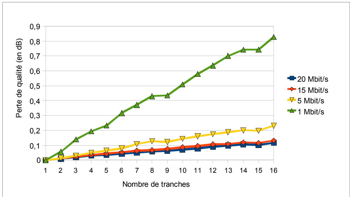
Figure 4.3 Perte de qualité, en dB, de l'approche originale d'Intel en fonction du nombre de tranches pour des débits de 1, 5, 15 et 20 Mbit/s.
