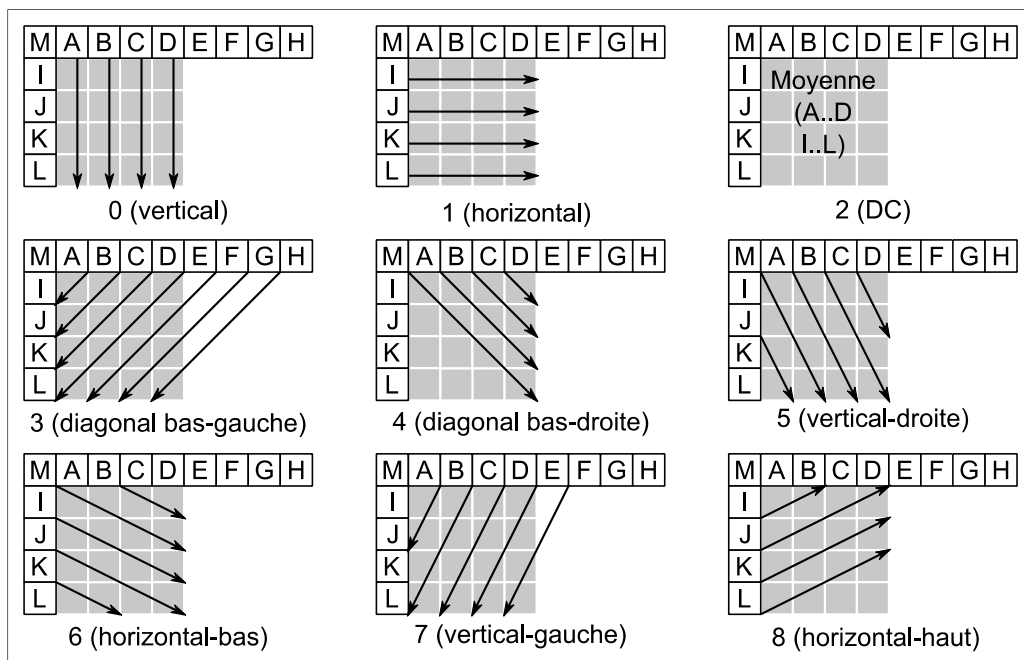
Figure 2.7 Modes de prédiction intra pour des blocs Y 4 \times 4 .
