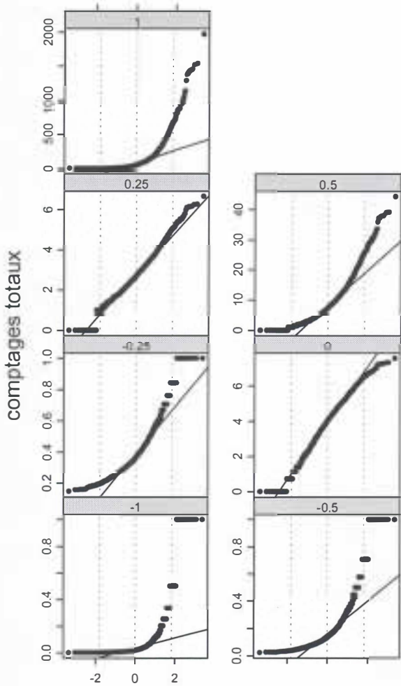
quantiles de la loi normale
