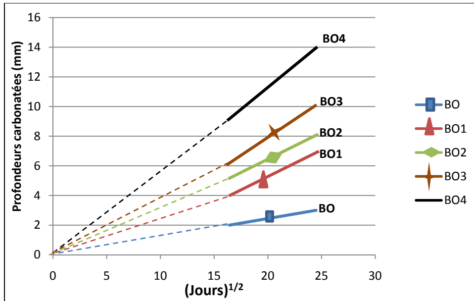
Figure 3.17 Profondeur de carbonatation mesurée par projection de phénolphthaleïne sur les bétons d'étude (exposition naturelle)
