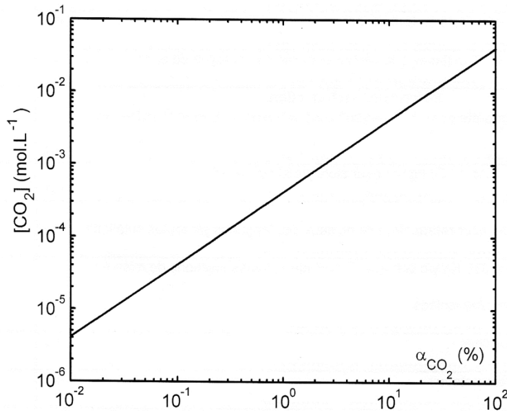
Figure 1. 1 Concentration en \text{CO}_2 dans la phase gazeuse en fonction de la fraction volumique \alpha_{\text{CO}_2} (à 20° C et sous une pression atmosphérique de 105 Pa) [Thiery, 2005]
