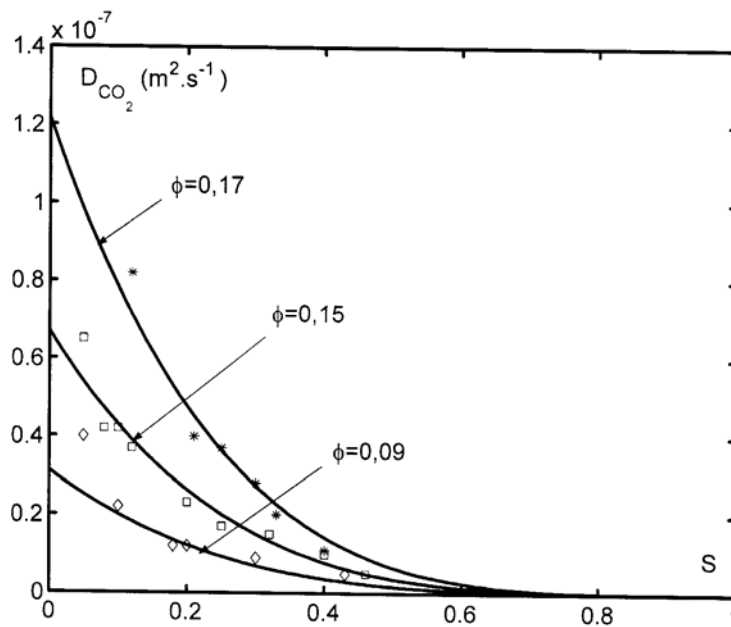
Figure 1. 37 Calage de la loi d'évolution du coefficient de diffusion au CO_2 en fonction de la porosité \phi et du taux de saturation S [mesures sur mortiers tirées de Papadakis et col, 1991b]
