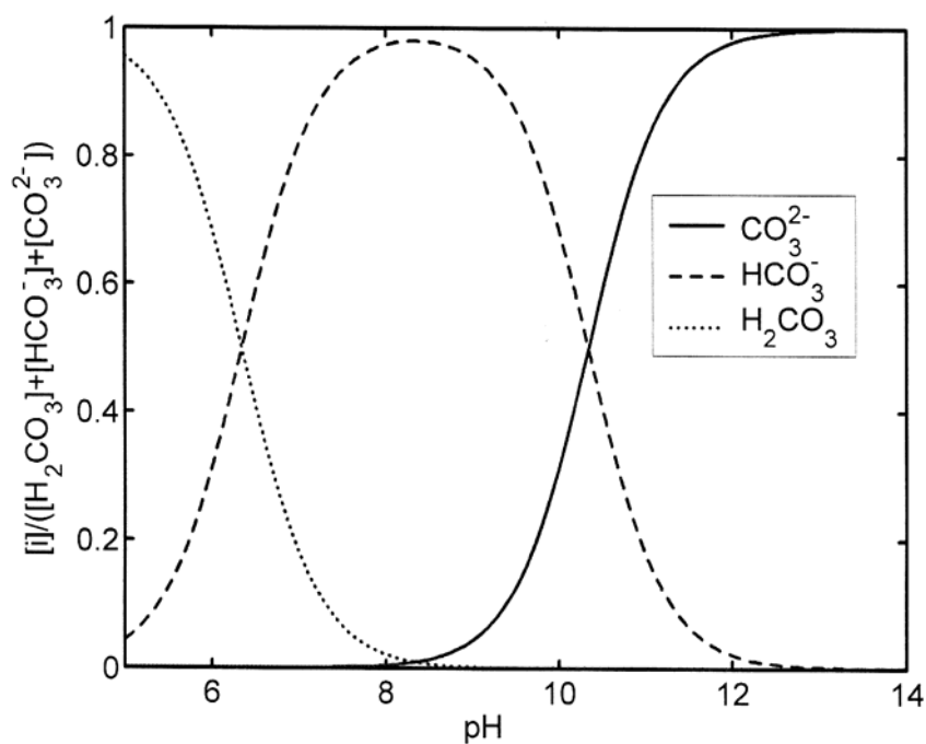
Figure 1. 2 Concentration du système des carbonates ( \text{H}_2\text{CO}_3 , \text{HCO}_3^- et \text{CO}_3^{2-} ) en fonction du pH (à 20^\circ \text{C} et à l'équilibre) (Thiery, 2005)
