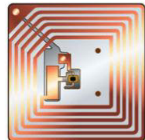
FIG 1.6 : Tag RFID actif.[10]
