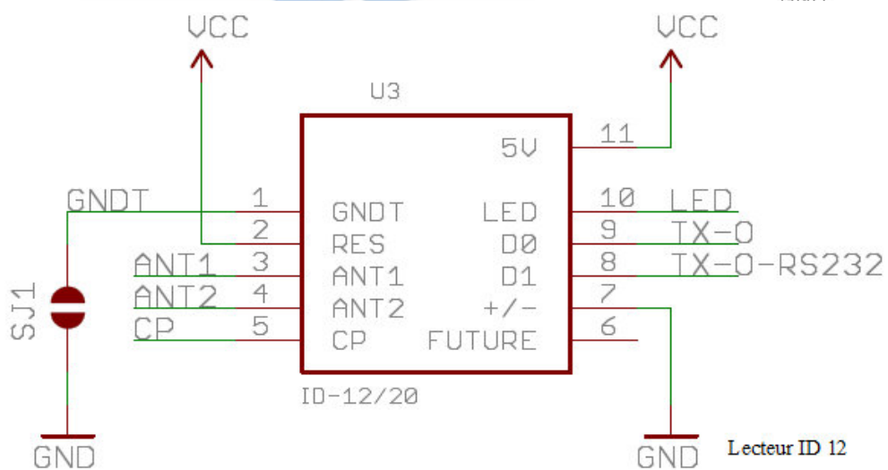
FIG 2.4 : Schéma électrique global du lecteur RFID. [14]
