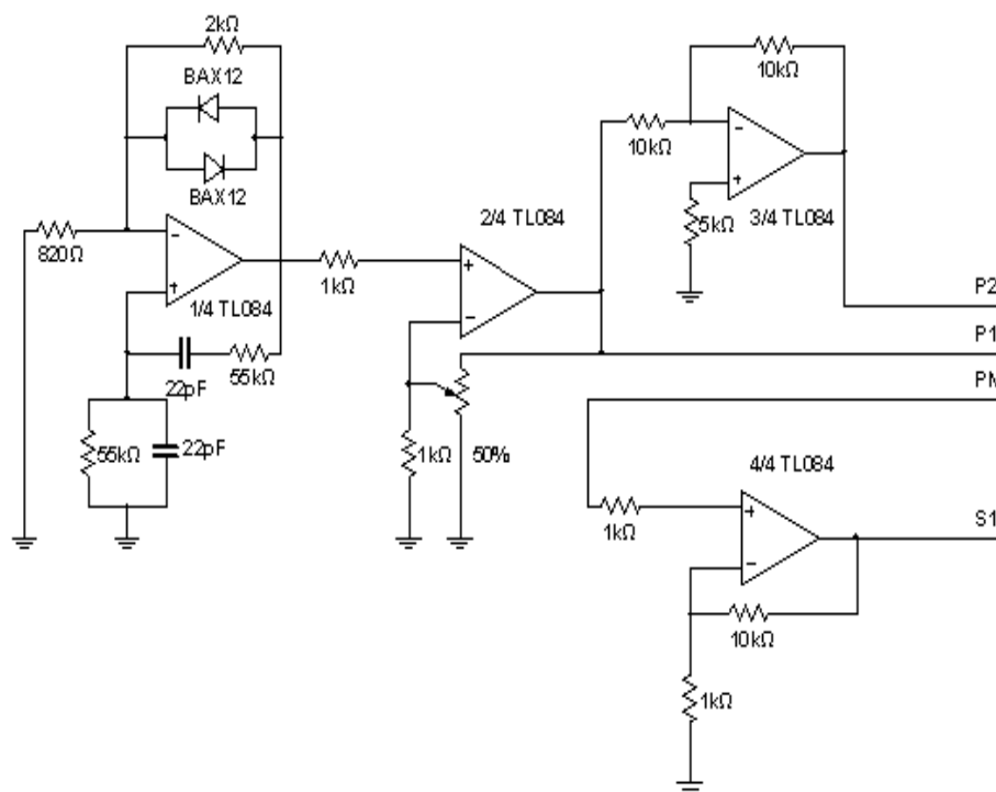
Figure 20 : Circuit oscillateur
