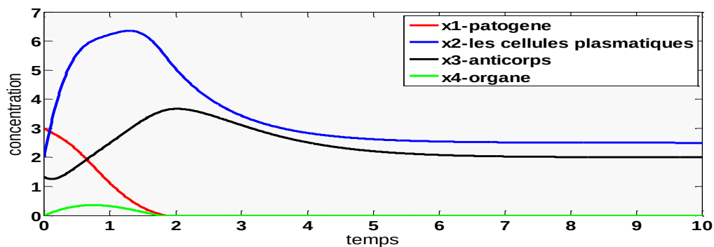
Figure 20: Equations d'états du système
