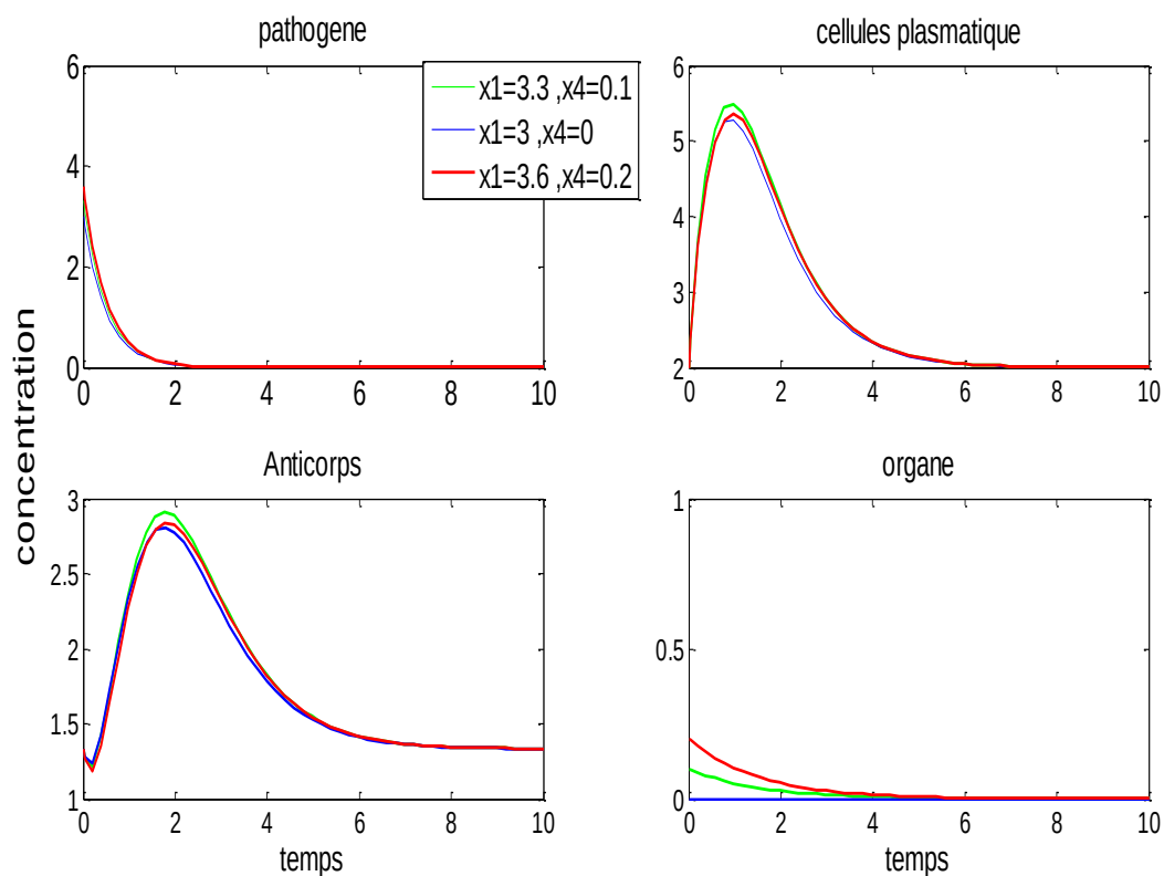
Figure 16: Trajectories de l'état de patients ayant des valeurs de paramètres perturbées.
