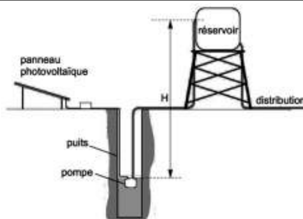
Schéma simplifié de l'installation
