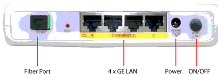
Figure 5 ONT
