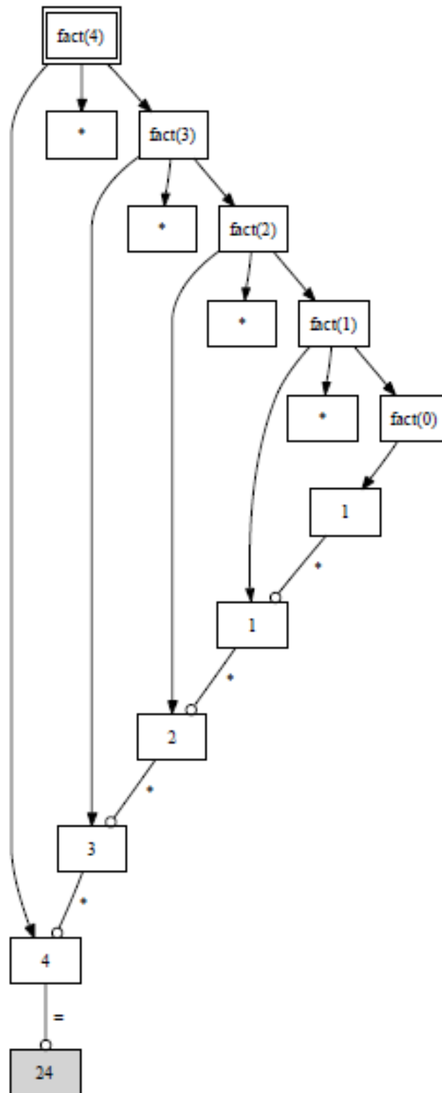
FIGURE 8.1 – Empilage/dépilage de 4!
