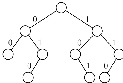
FIG. 12 – Le code de l'arbre est \{\varepsilon, 0, 1, 00, 01, 10, 11, 010, 101, 110\} .
