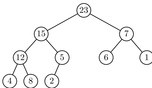
FIG. 16 – Un arbre tassé.
