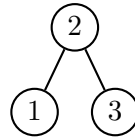
FIG. 9 – L'arbre produit par la suite d'insertions 2, 1, 3, ou par la suite 2, 3, 1.
