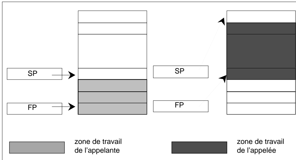
Figure 4.19: Principe de la pile d'exécution
