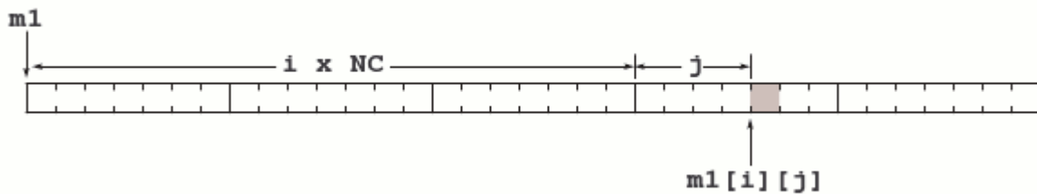
Fig. 10 - Tableau bidimensionnel statique
