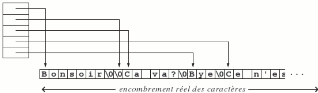
Fig. 14 - Tableau de chaînes de caractères
