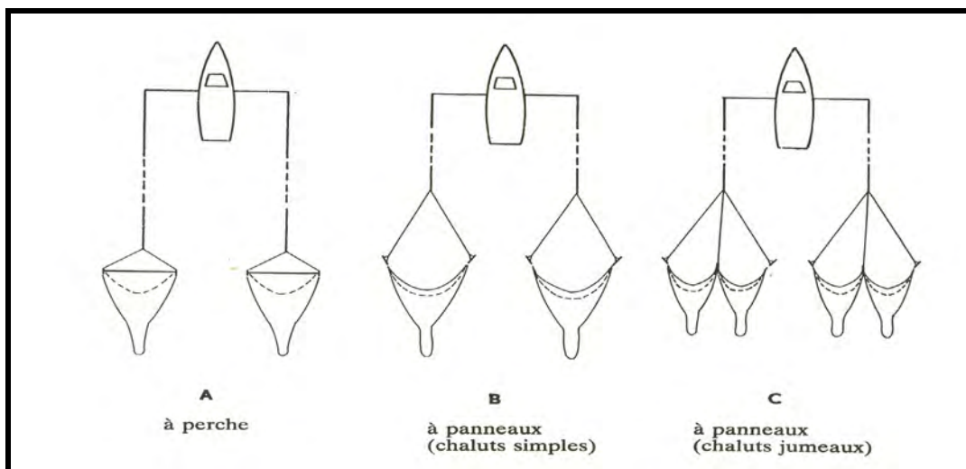
Figure 11 : Chaluts de fond de capture de crevettes, à faible ou moyenne ouverture verticale et à grand développement horizontal (Source : catalogue des engins de pêche/ IFREMER)
