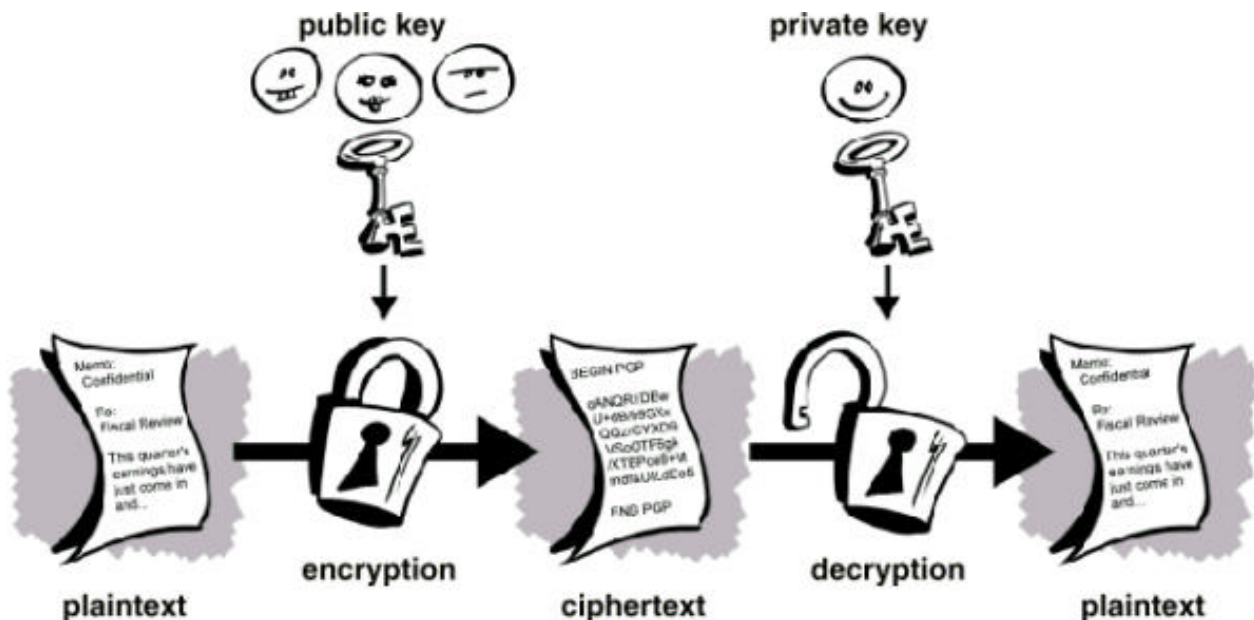
Figure 3-1. Diagramme de la cryptographie à clé publique
